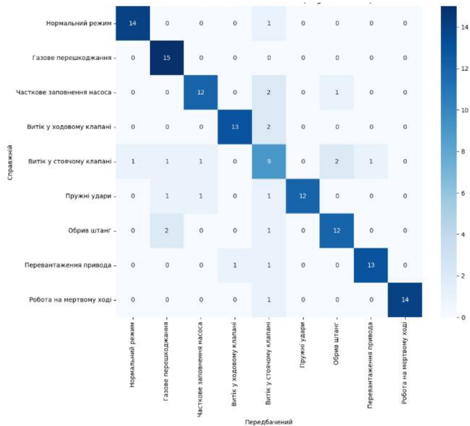
Рисунок 2 – Результати валідування роботи моделі
