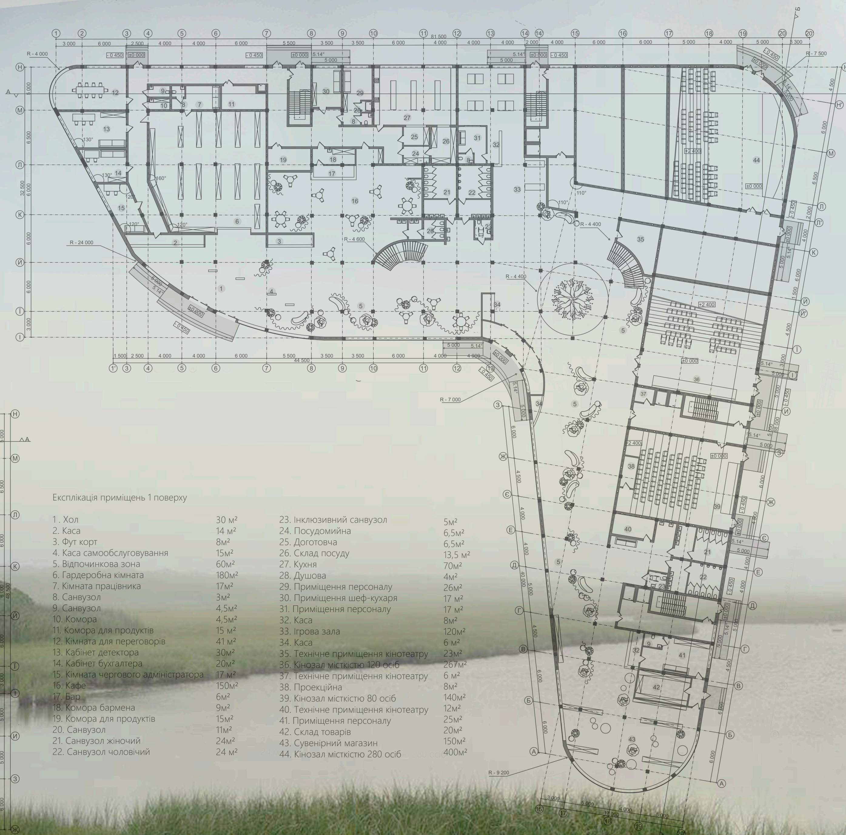
План 1 поверху М 1: 250 на відмітці +2 400
