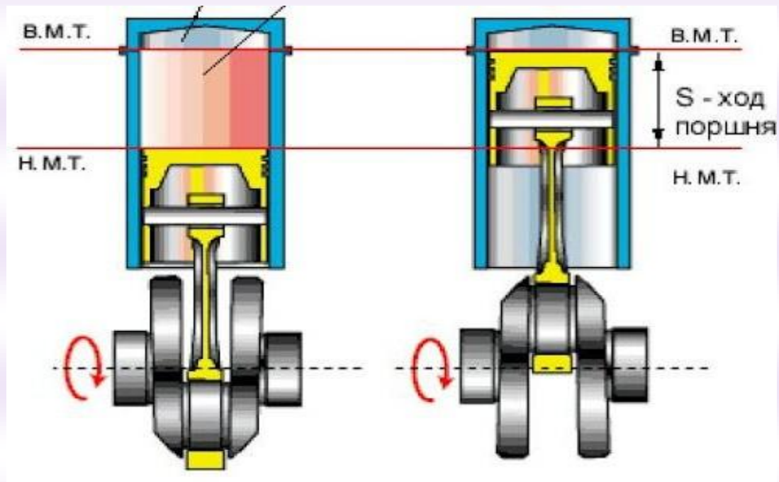
Рисунок 9.2 – Визначення вакууму в циліндрі двигуна
