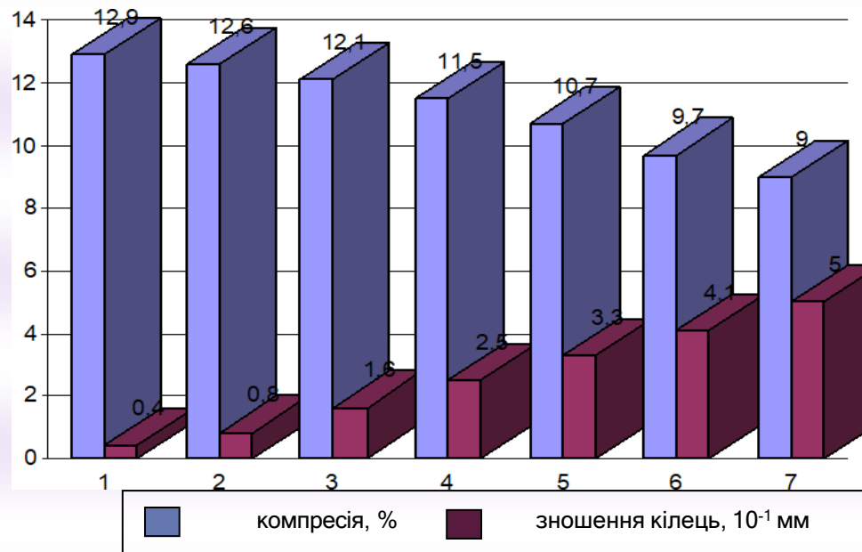
Рисунок 14.2 – Співвідношення між зниженням компресії та зносом поршневих кілець у мм
