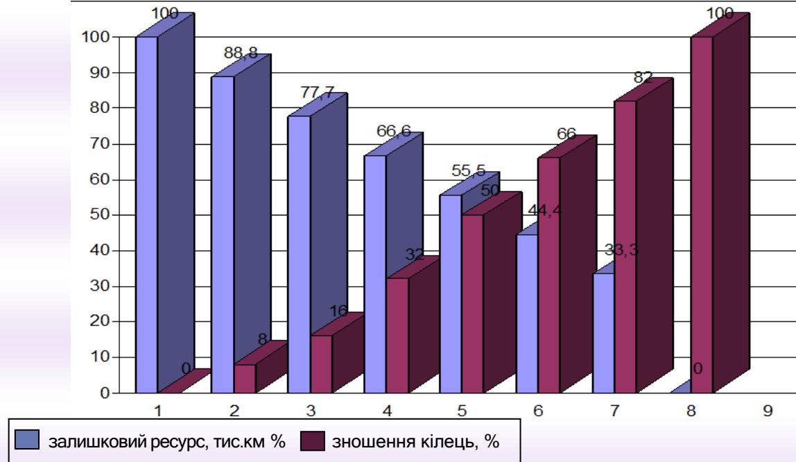
Рисунок 15.1 – Співвідношення між залишковим ресурсом та зношенням поршневих кілець у %
