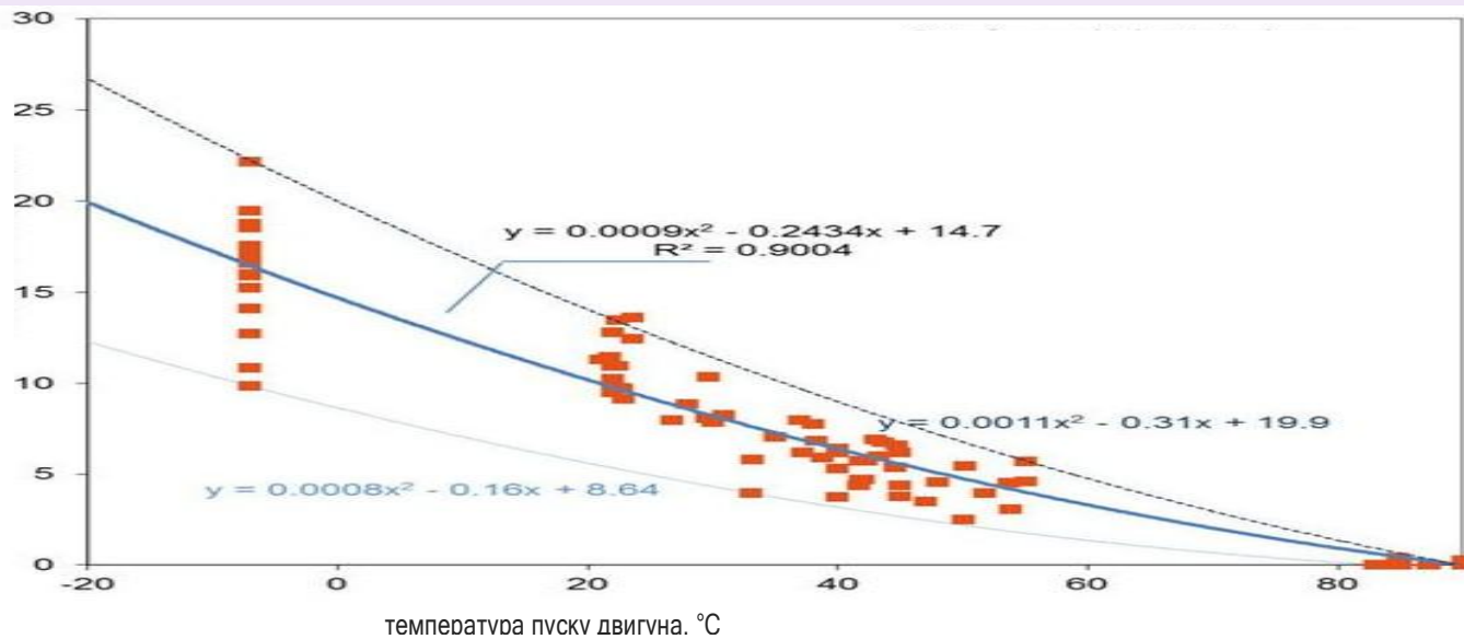
Рисунок 5.1 – Зміна витрати пального залежно від температури навколишнього середовища
