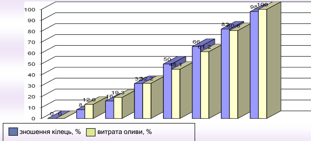
Рисунок 14.1 – Співвідношення між витратою оливи та зносом поршневих кілець у %
