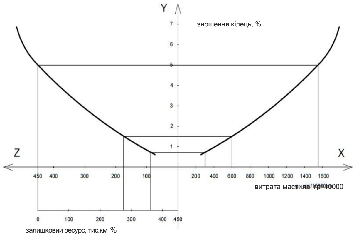
Рисунок 3.11 – Номограма зміни витрати оливи, зношення поршневих кілець та залишкового ресурсу двигуна автомобіля Skoda Fabia
