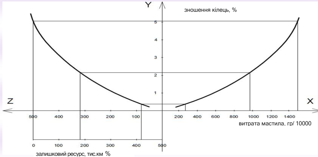
Рисунок 13.1 – Номограма зміни витрати оливи, зносу поршневих кілець та залишкового ресурсу двигуна автомобіля Dacia Logan
