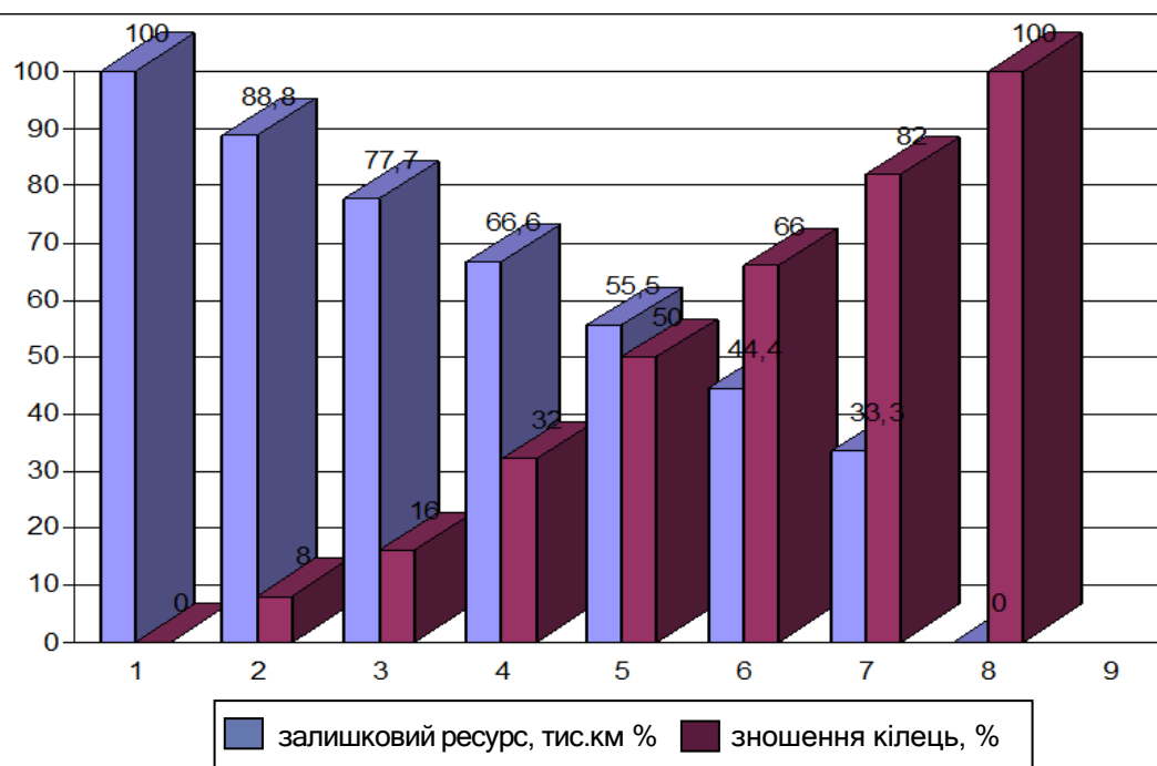
Рисунок 3.10 – Співвідношення між залишковим ресурсом та зношенням поршневих кілець у %
