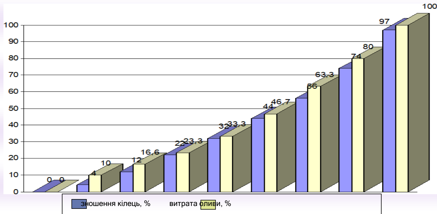
Рисунок 11.1 – Співвідношення між витратою оливи та зносом поршневих кілець у %
