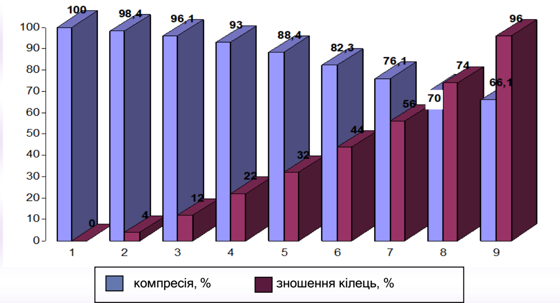
Рисунок 12.1 – Співвідношення між зниженням компресії та зносом поршневих кілець у %
