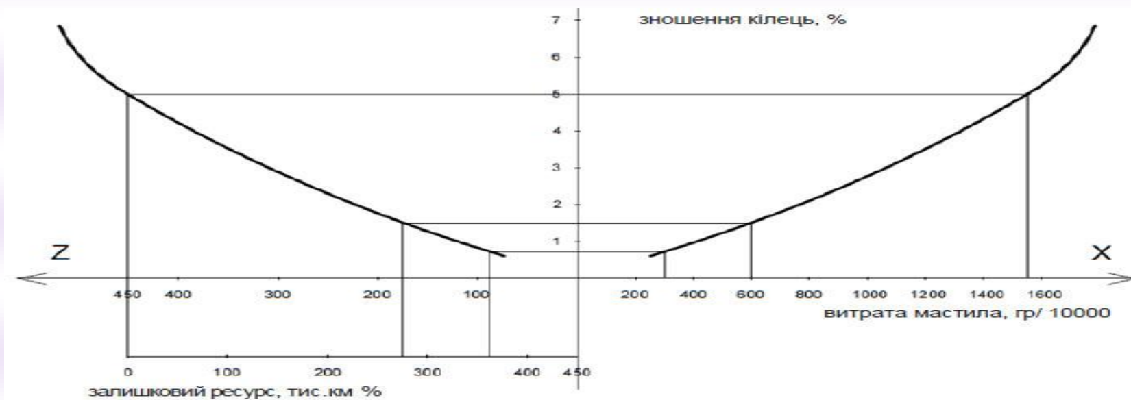
Рисунок 15.2 – Номограма зміни витрати оливи, зношення поршневих кілець та залишкового ресурсу двигуна автомобіля Skoda Fabia
