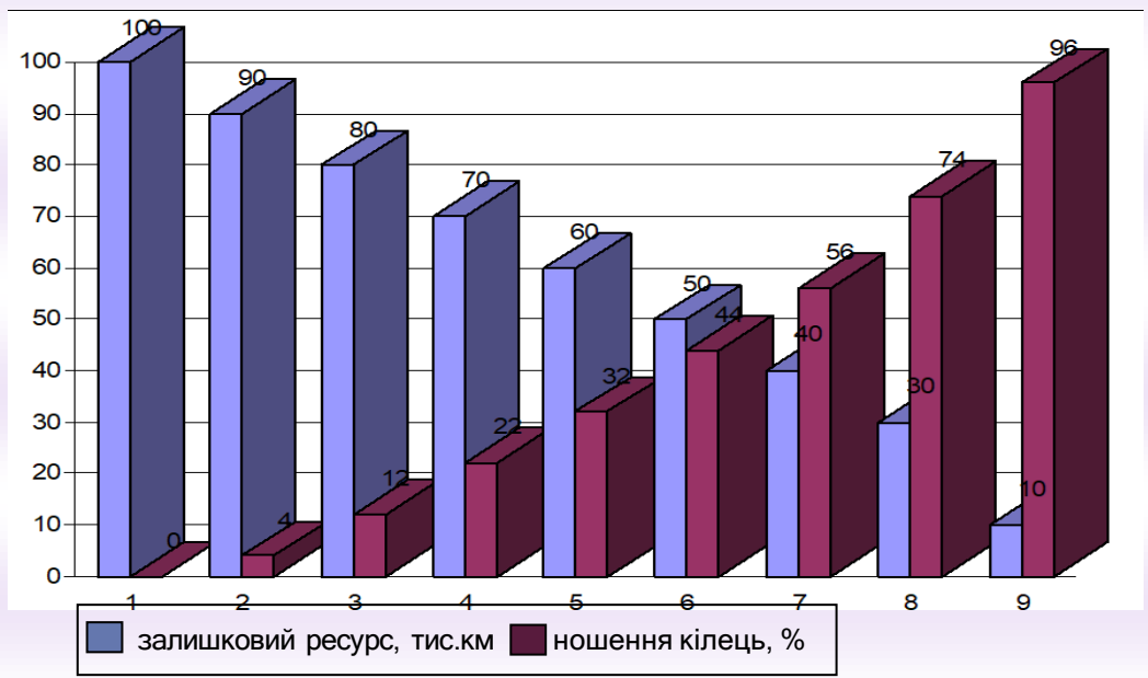
Рисунок 12.2 – Співвідношення між залишковим ресурсом двигуна та зношенням поршневих кілець у %
