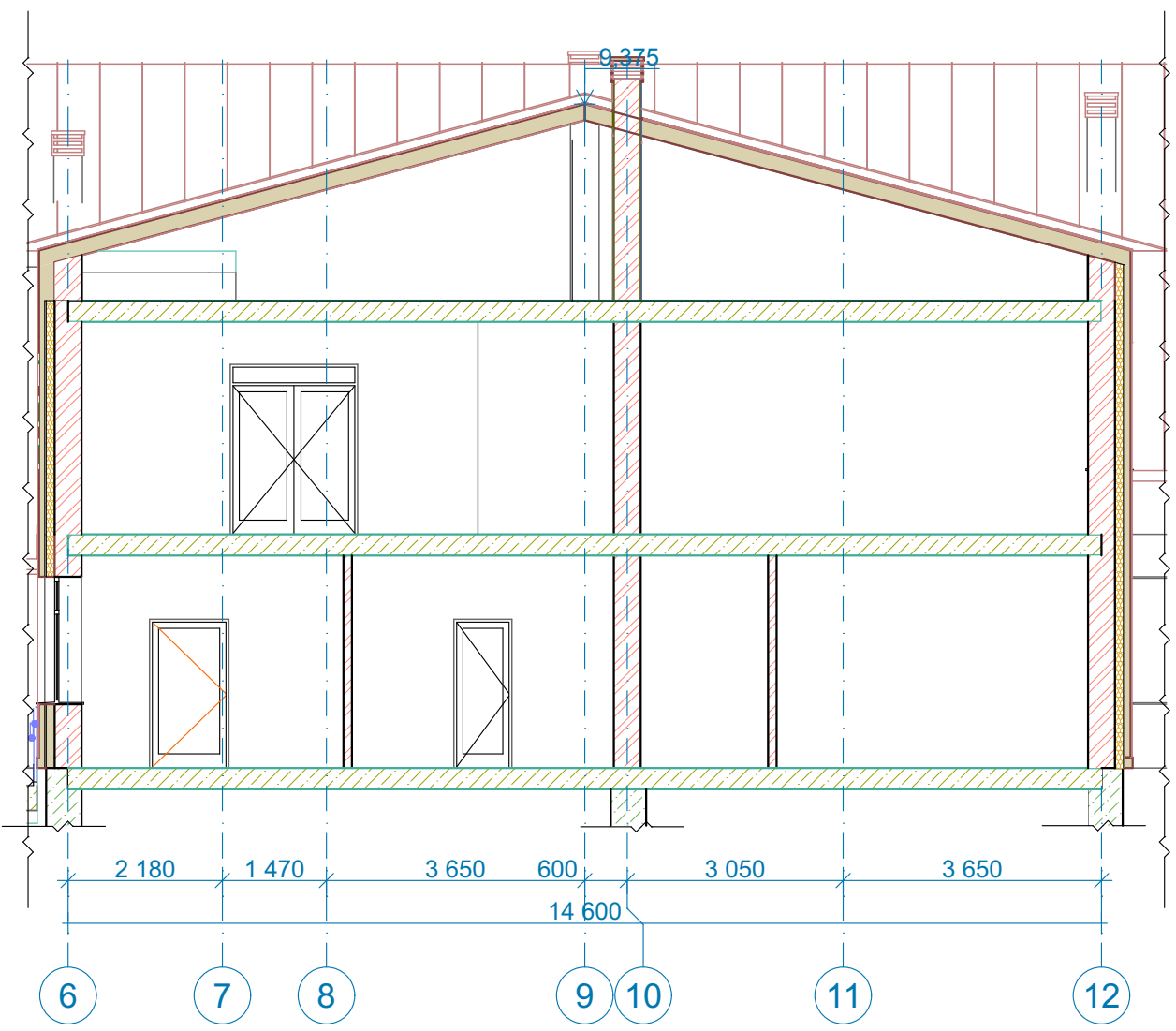
Розріз 8-8 в осях 6-12
