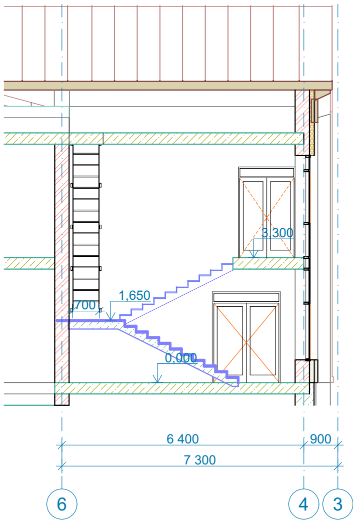
Розріз 2-2 в осях 6-3
