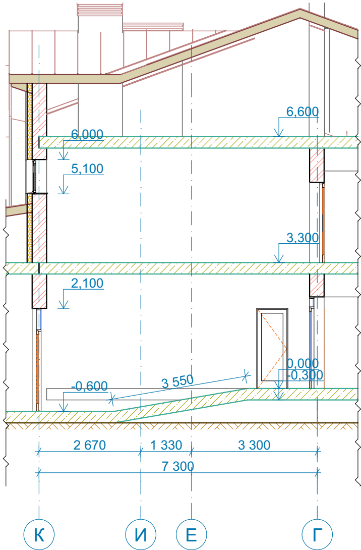
Розріз 7-7 в осях К-Г
