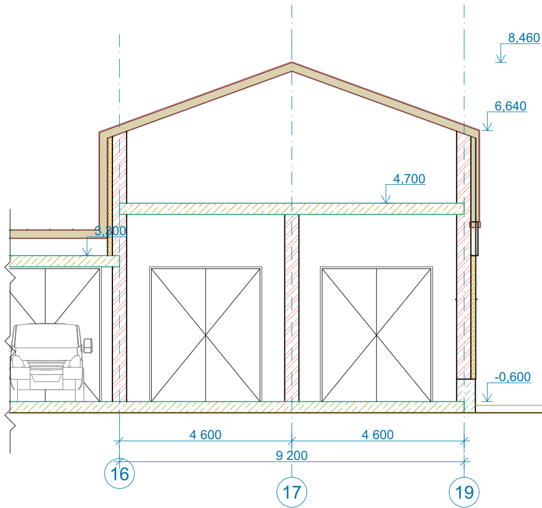
Розріз 3-3 в осях 16-19
