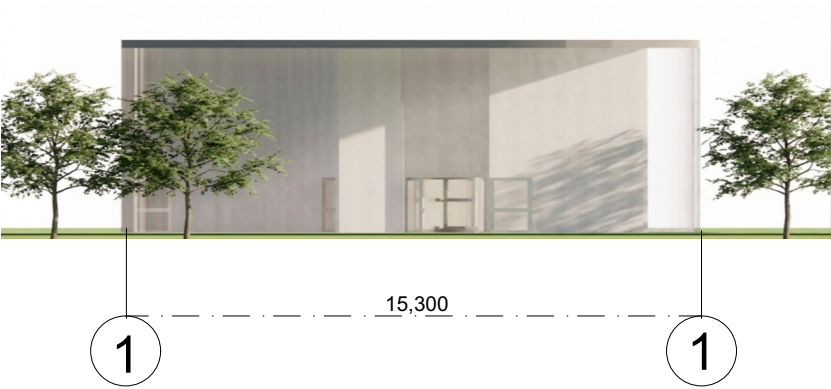
Фасад комерційного приміщення в осях 1-1 м 1:200
