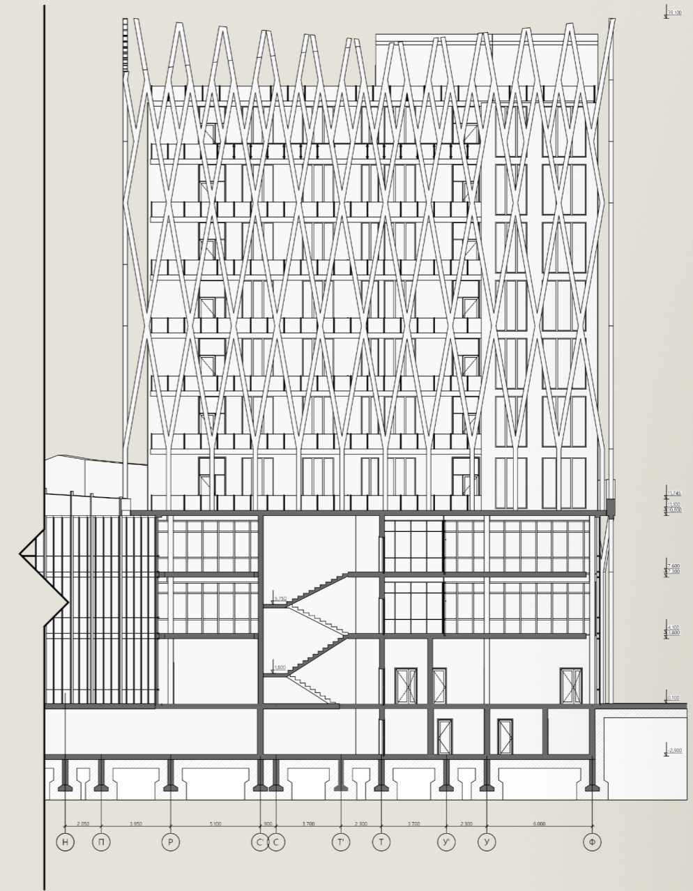
Розріз 2-2 М 1:250
