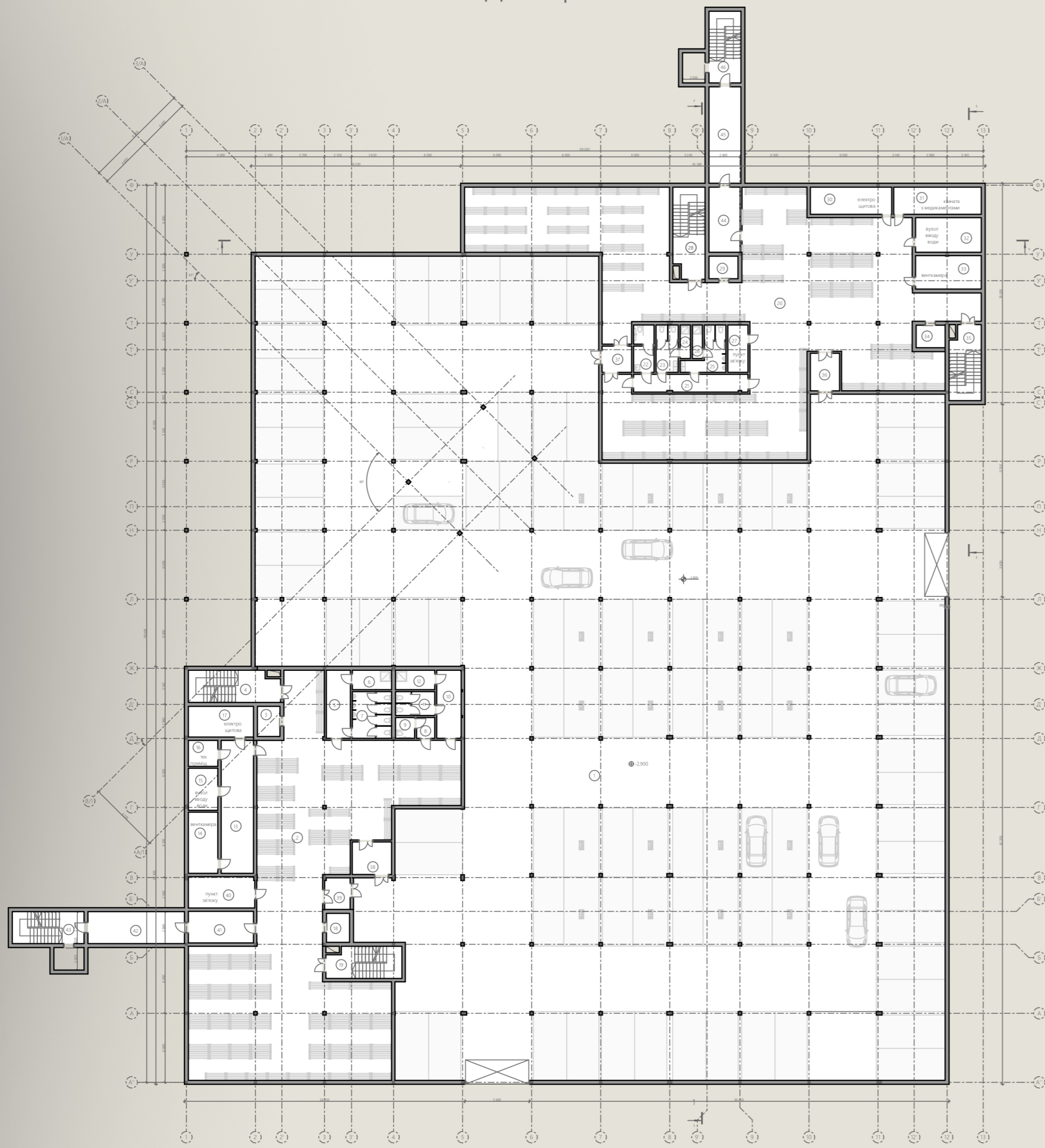
План на відмітці +0.150 М 1:250
