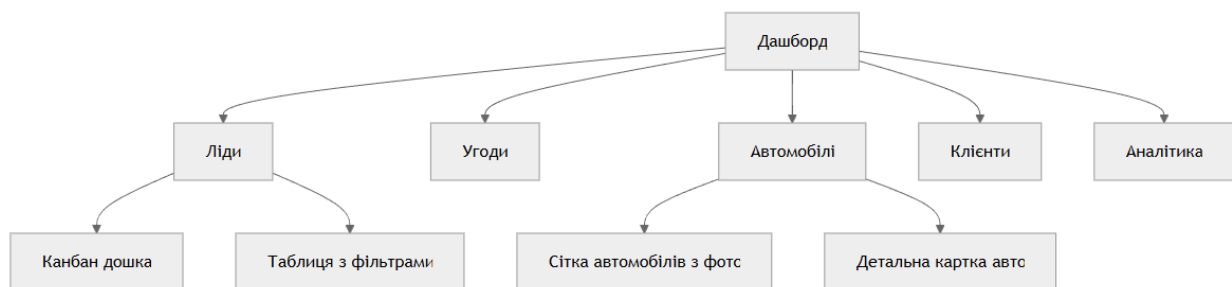
Рисунок 3.9 – Діаграма компонентів інтерфейсу
