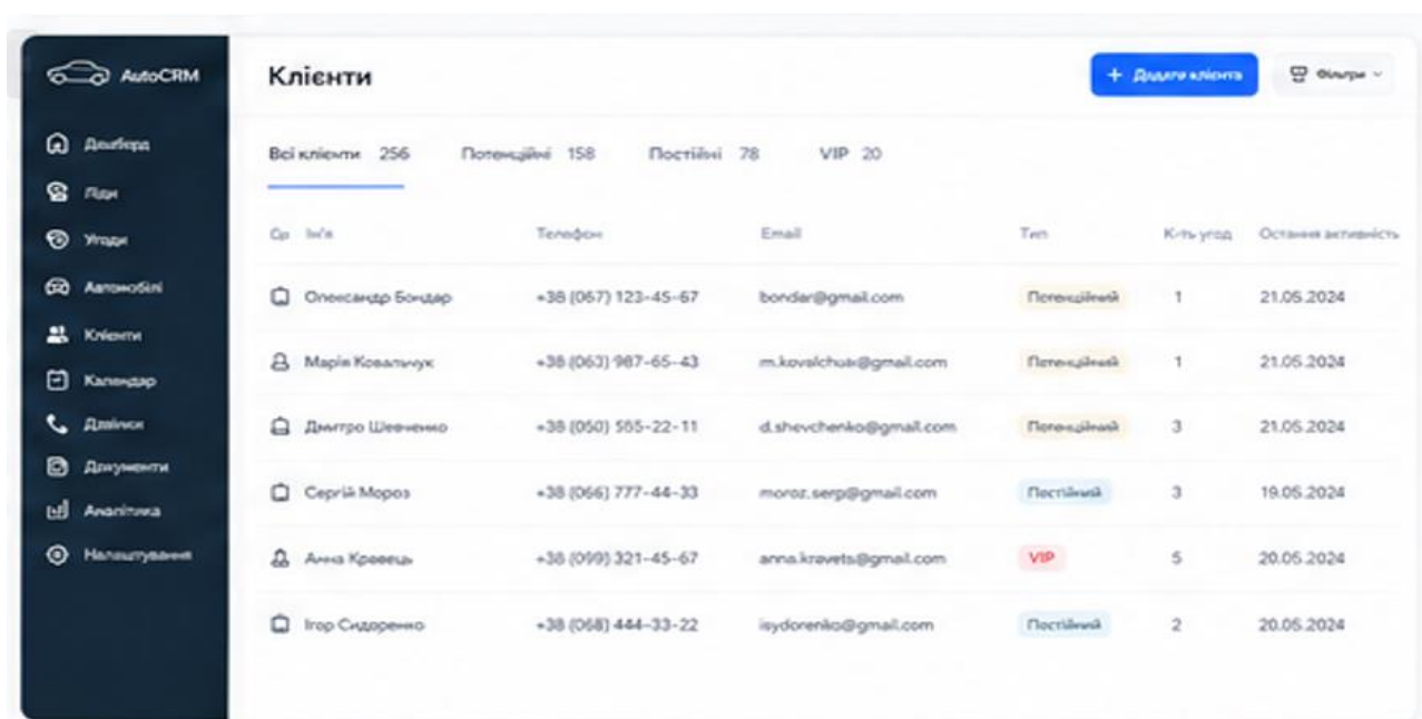
Рисунок 3.5 – Інформаційне меню клієнтів у CRM системі
