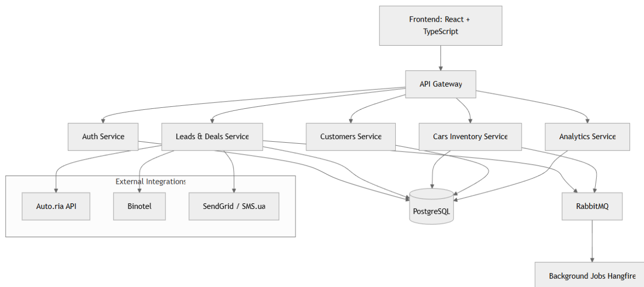
Рисунок 3.7 – Діаграма архітектури системи
