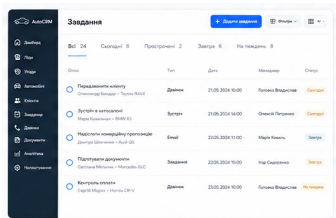
Рисунок 3.6 – Меню списку завдань в CRM системі
