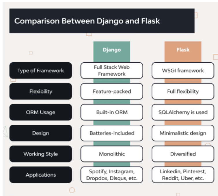
Рисунок 1.9 – Наглядне порівняння фреймворків Django та Flask [13]
