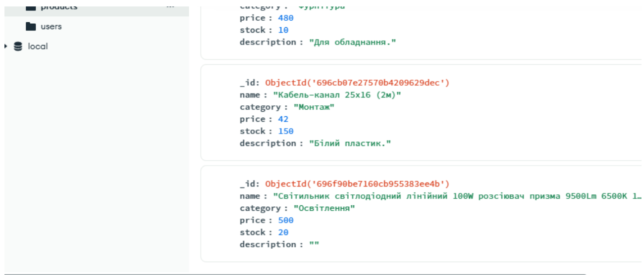
Рисунок 4.33 – Вигляд колекції “products” в базі даних “electrical_db” на сайті ПЗ MongoDB Atlas
