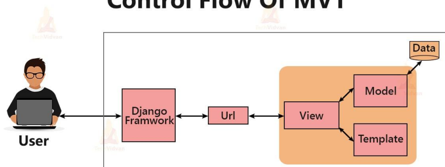
Рисунок 1.6 – Архітектура Django MVT (Model-View-Template) [12]
