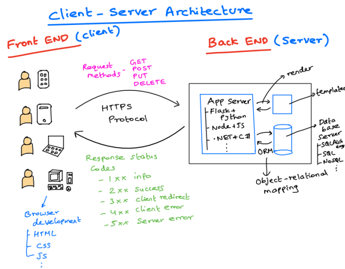
Рисунок 2.1 – Архітектура «Клієнт-Сервер» [23]
