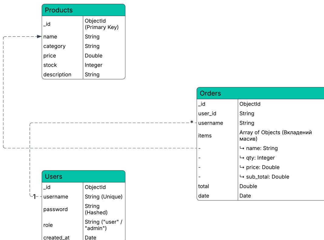
Рисунок 2.2 – Структурна схема бази даних додатку “electro_advisor”
