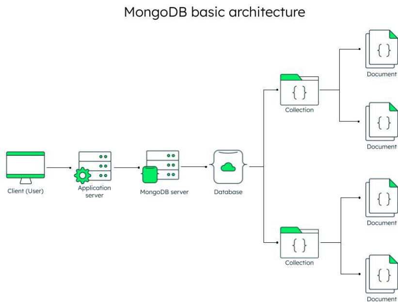
Рисунок 1.10 – Базова архітектура MongoDB [19]
