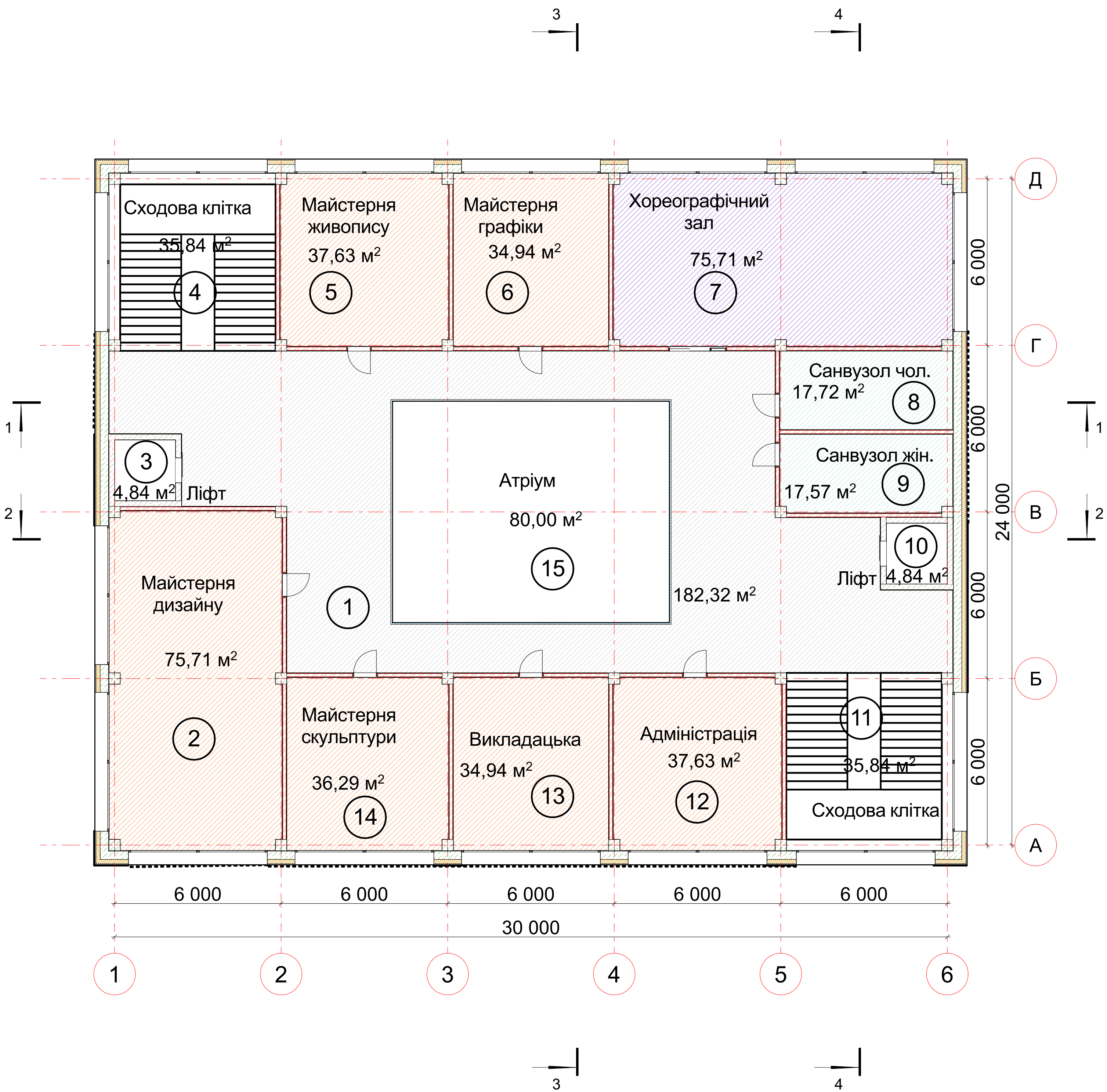
План другого поверху 1:100
