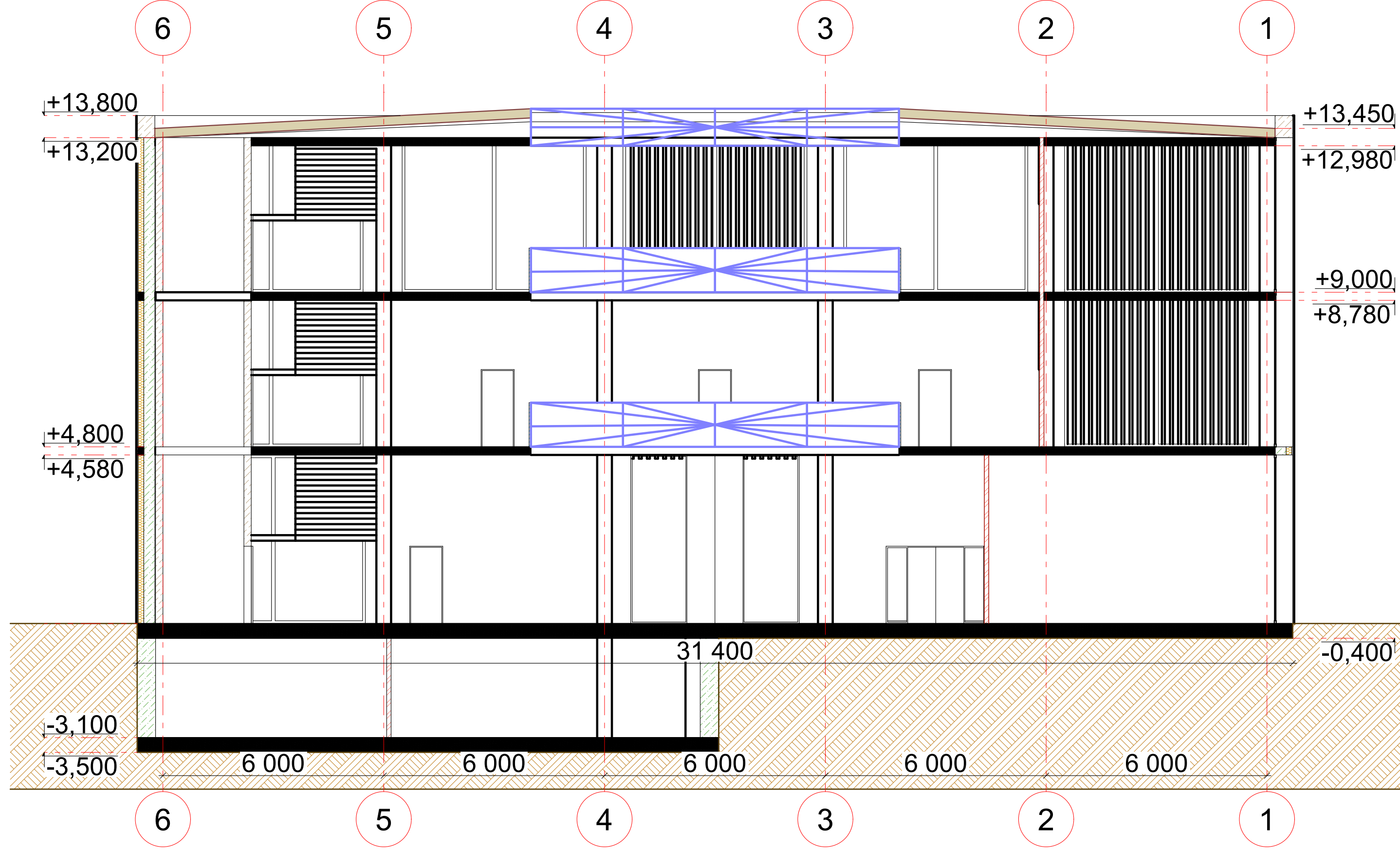
2-2 1:100
