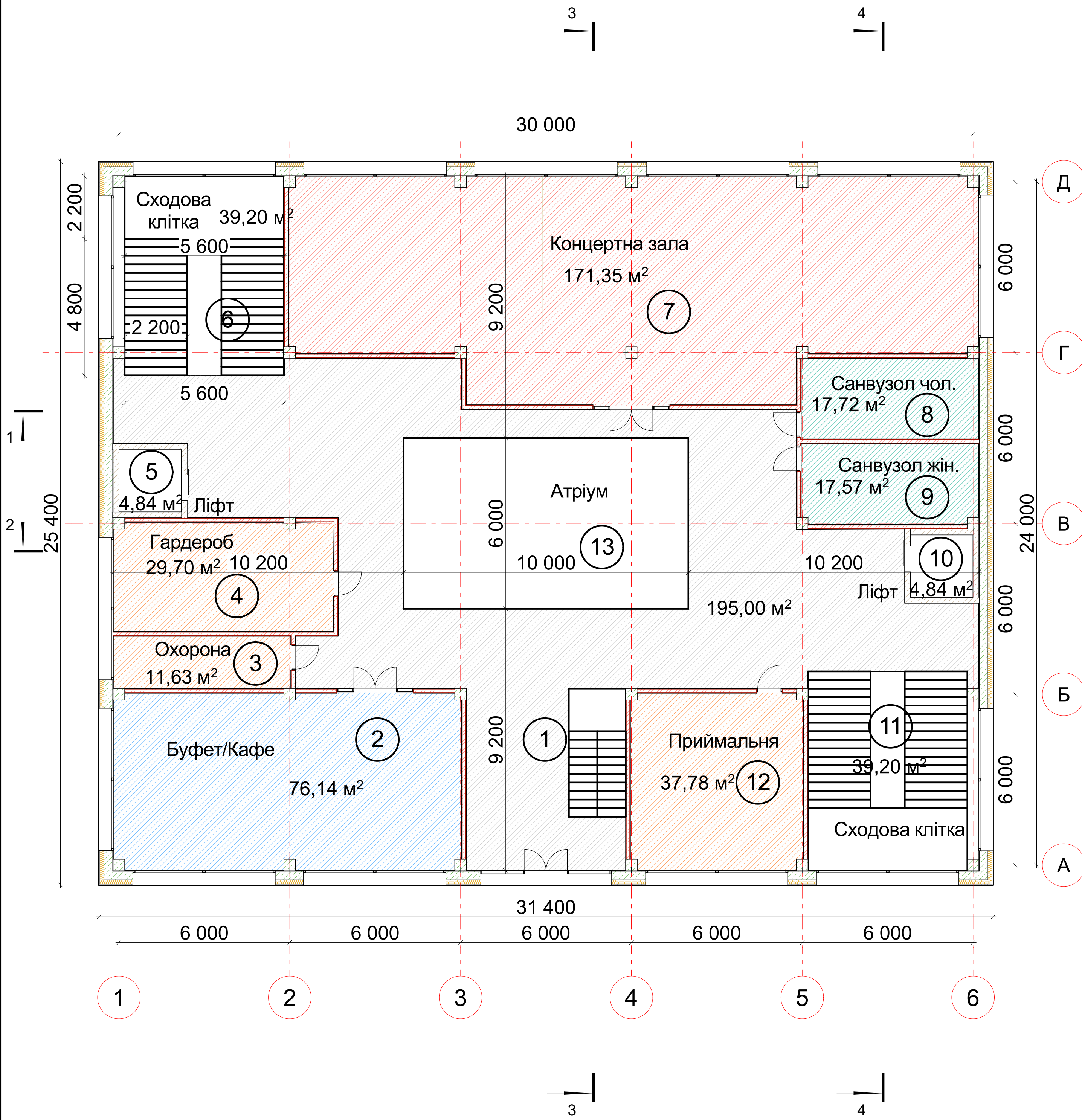
План першого поверху 1:100
