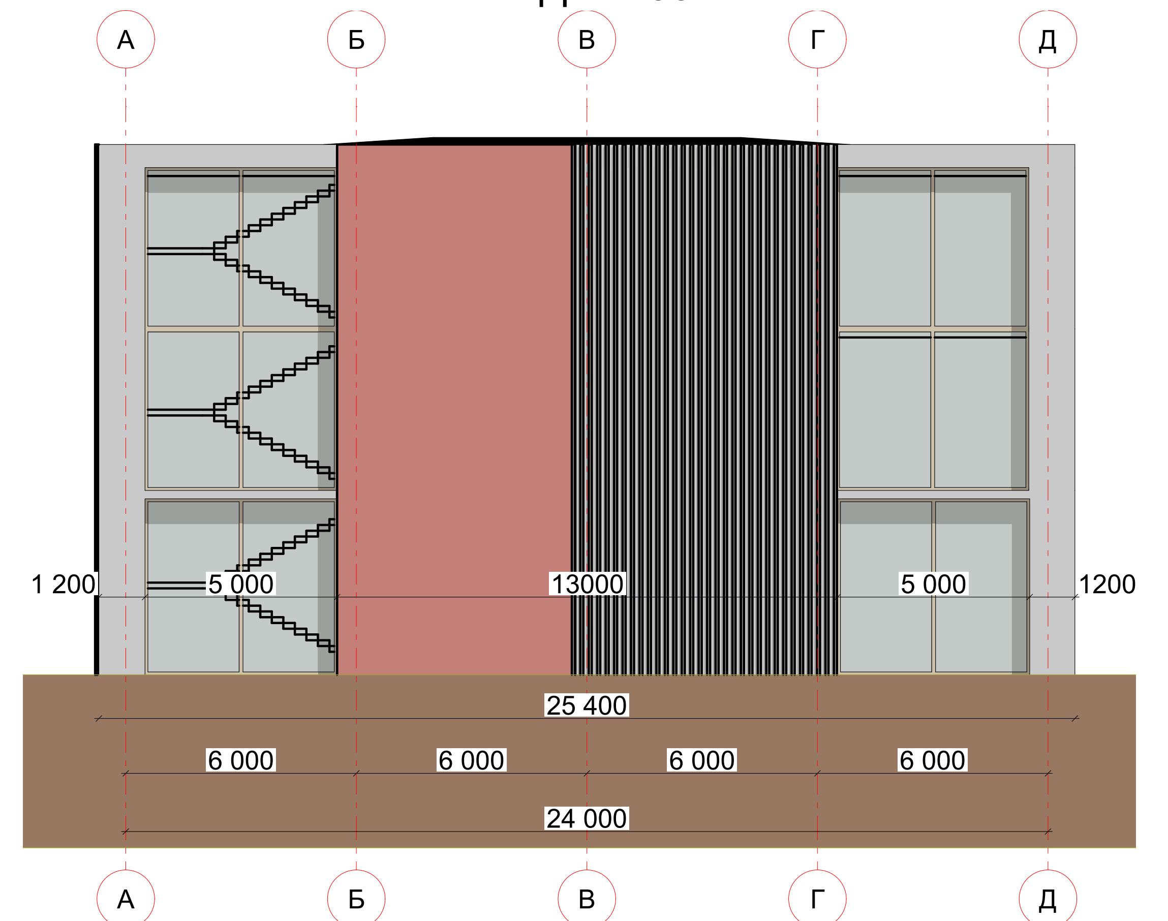
А-Д 1:100
