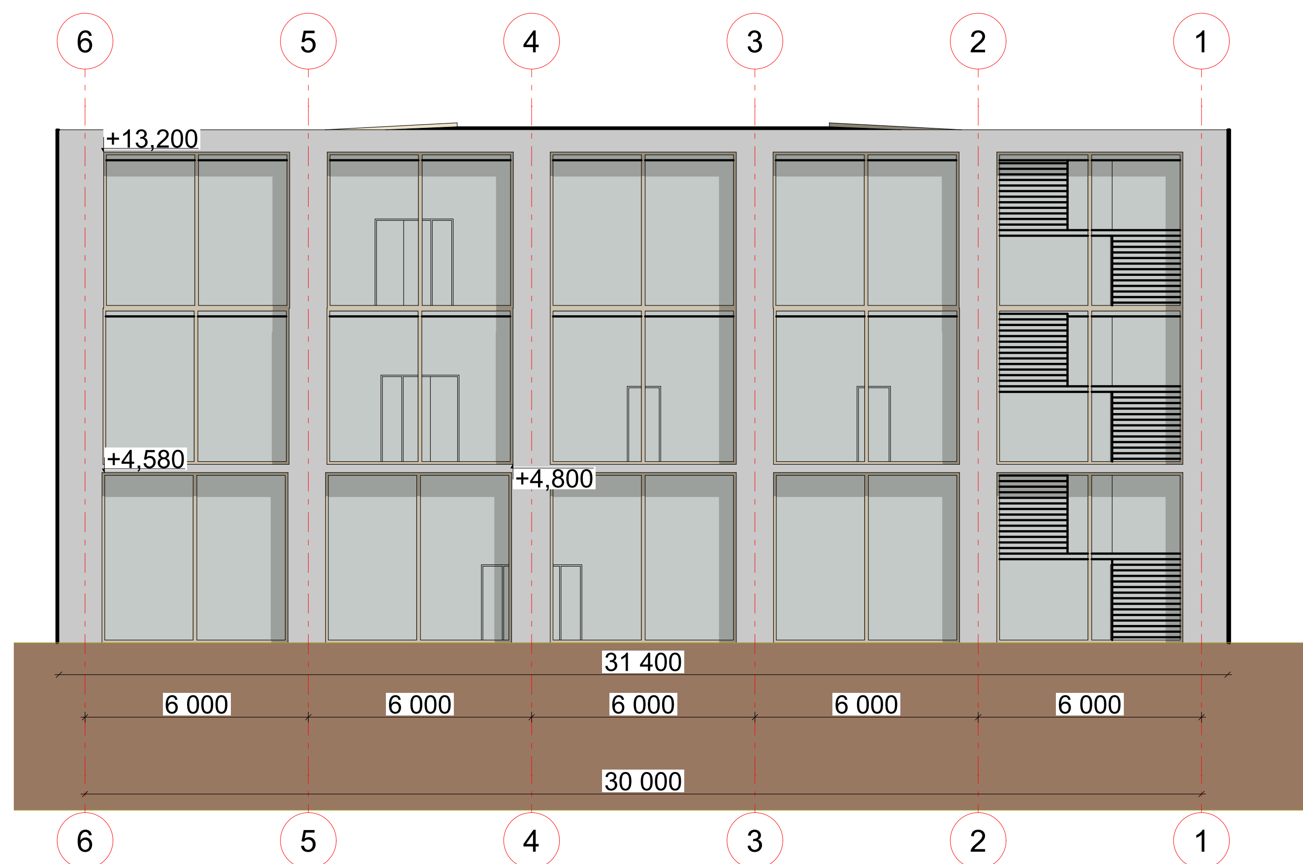
6-1 1:100
