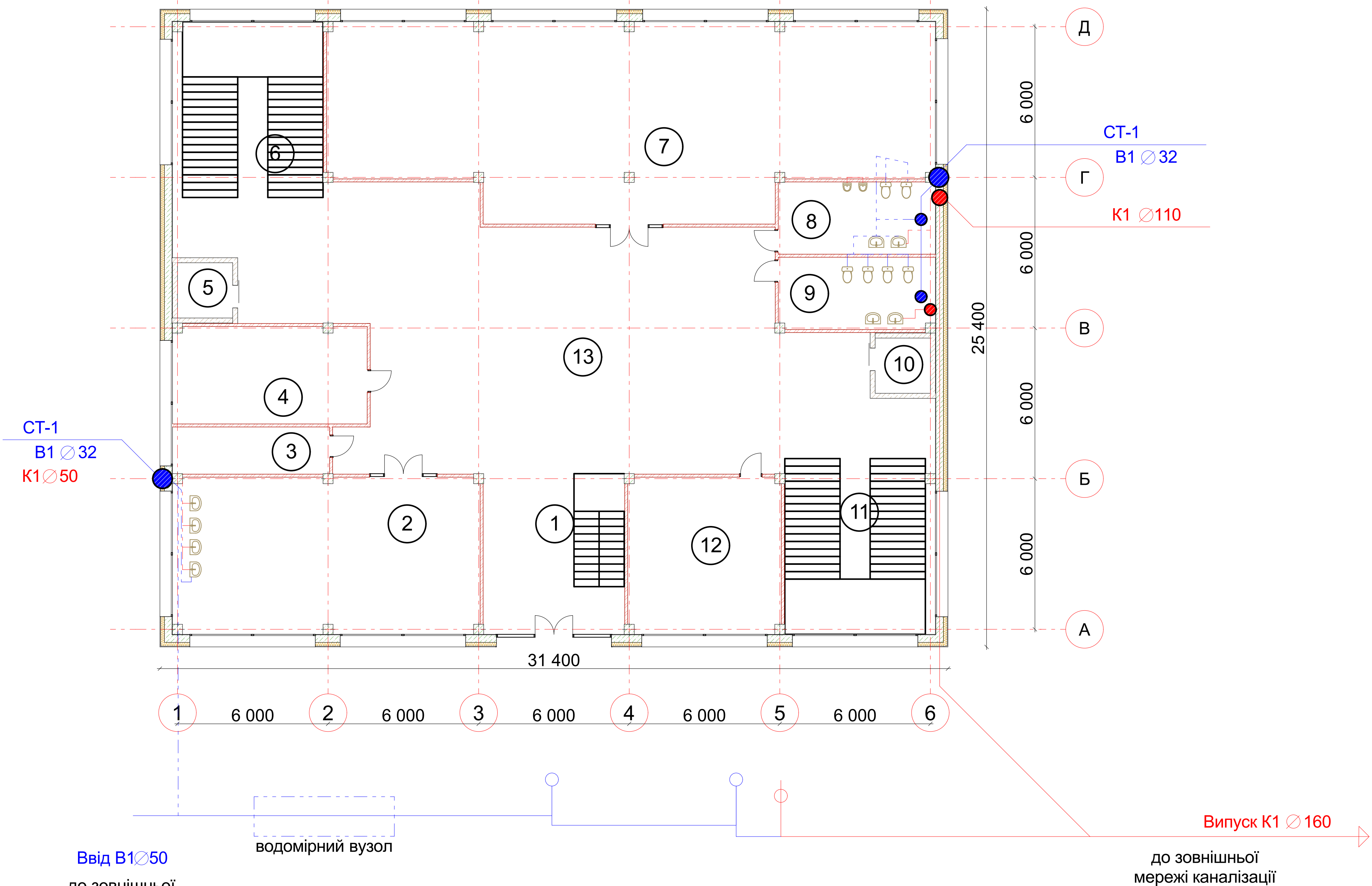
Схема першого поверху 1:100
