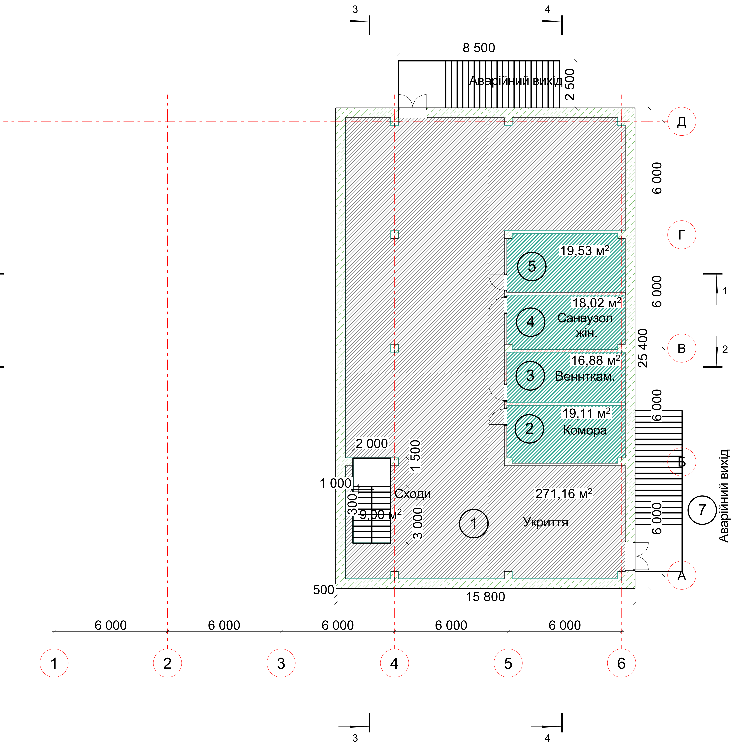
План укриття 1:100
