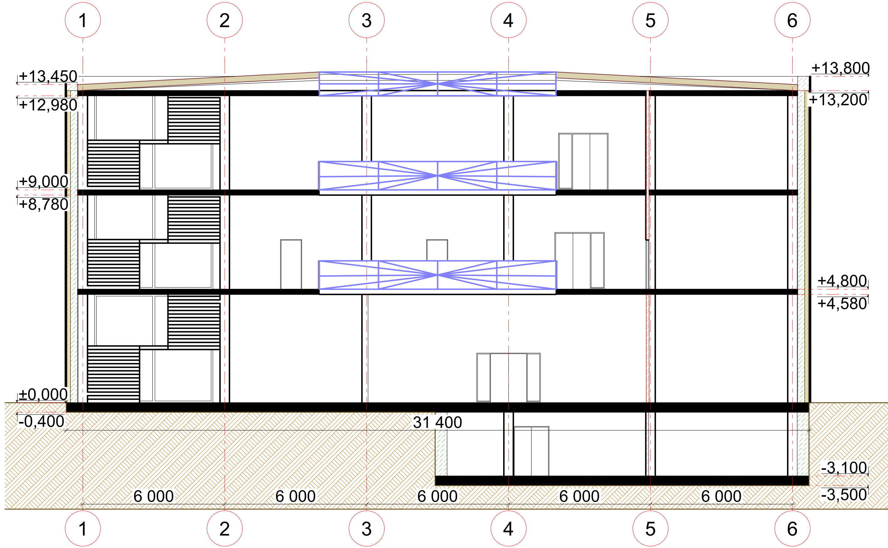
1-1 1:100
