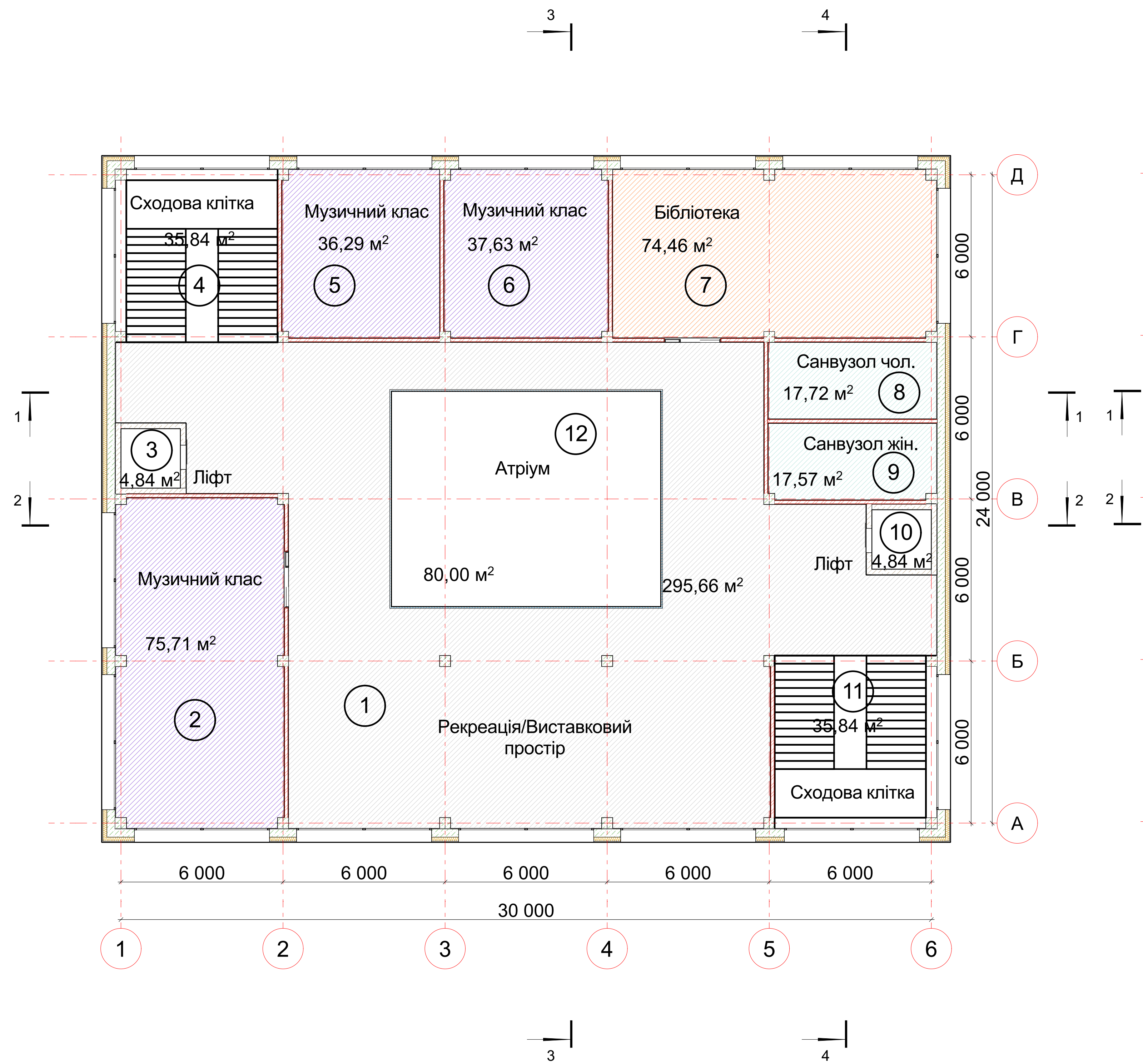
План третього поверху 1:100
