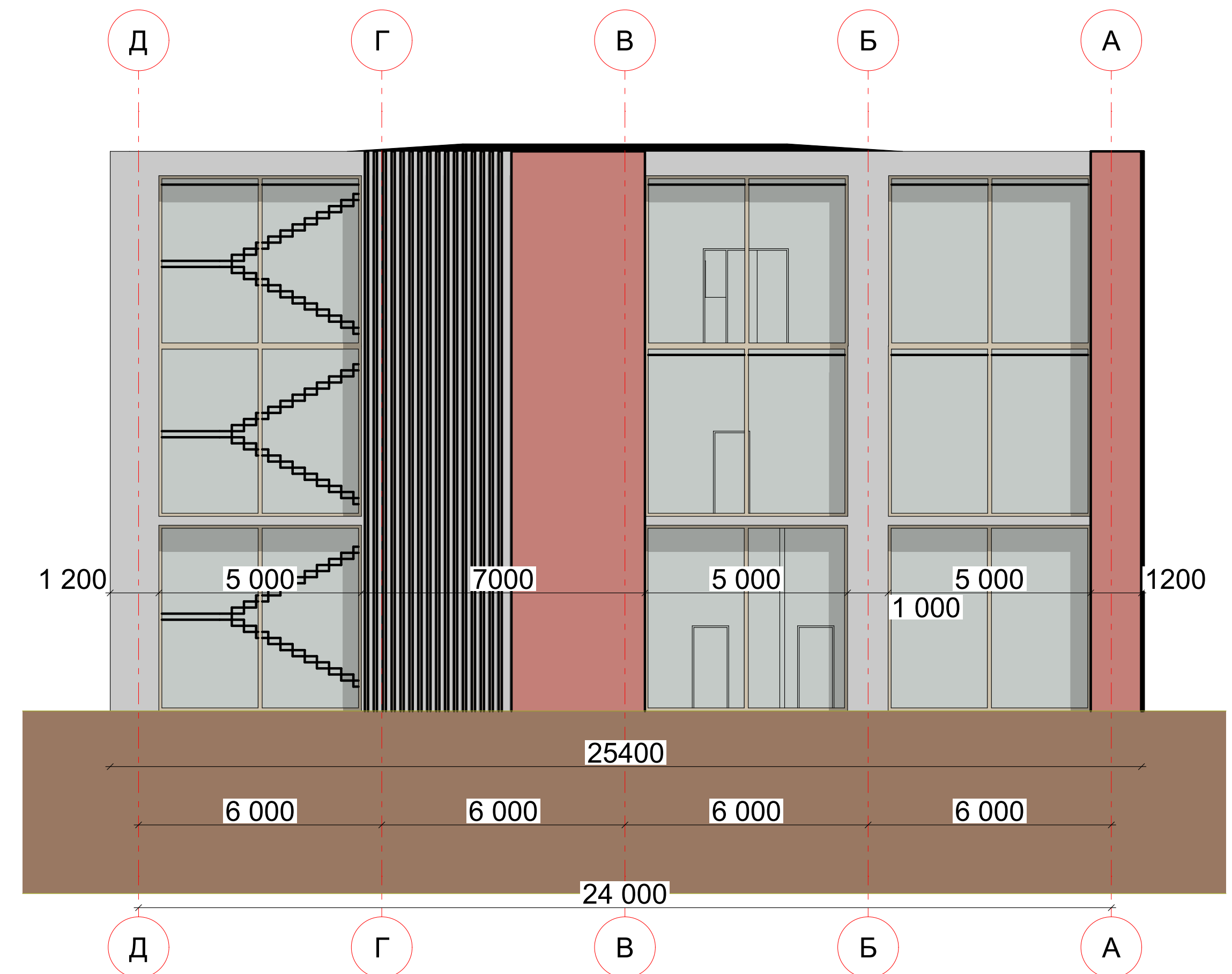
А-Д 1:100
