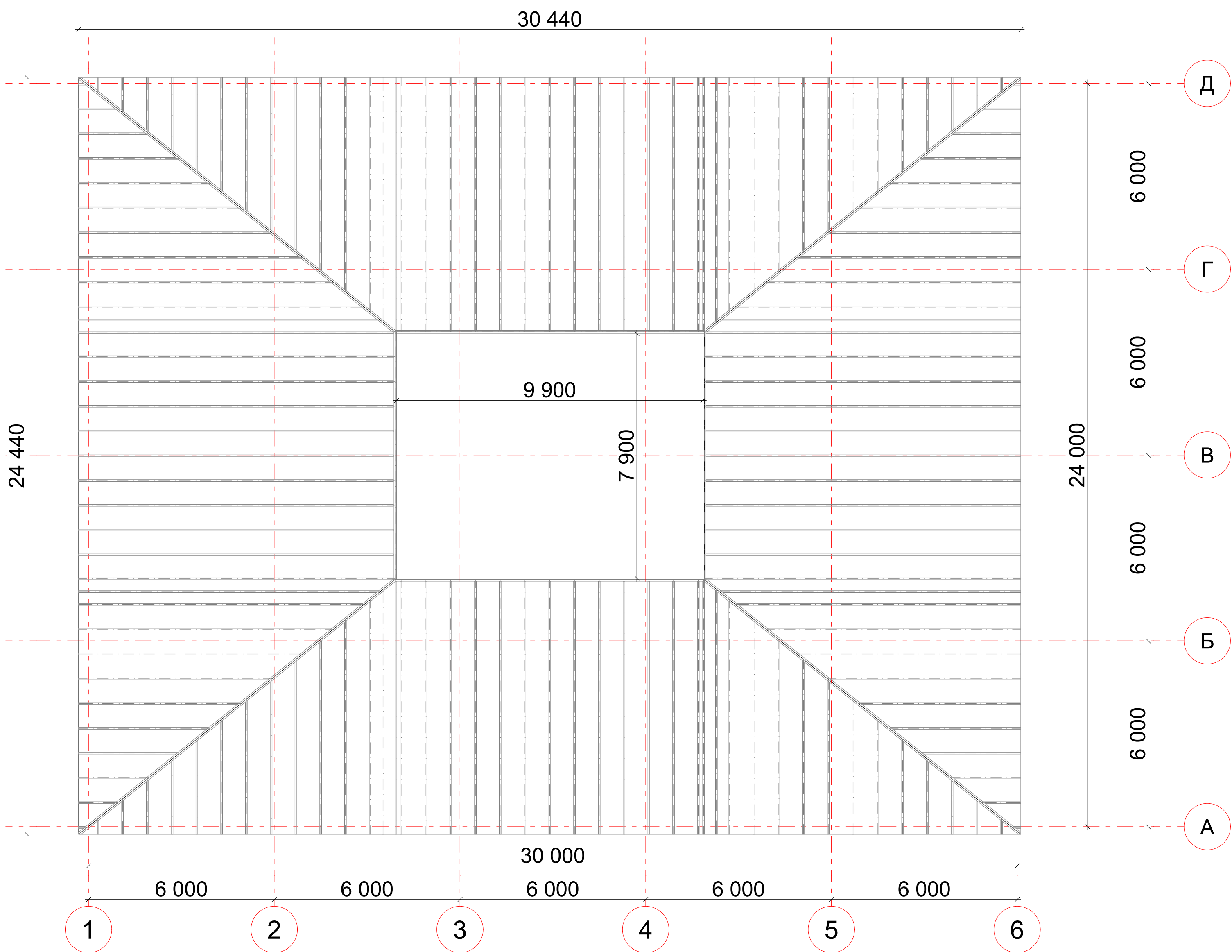
Схема крокв 1:100
