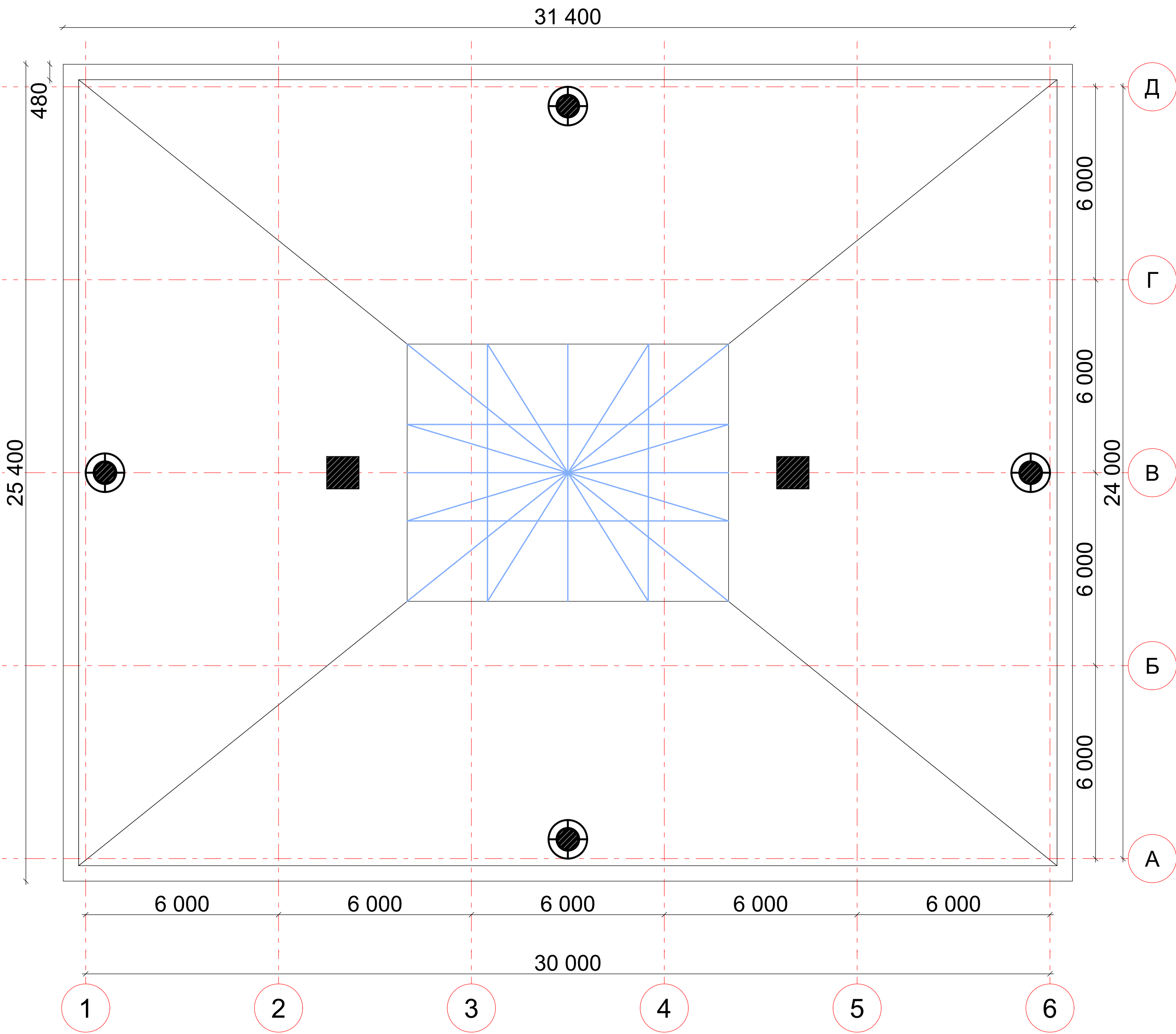
Схема покрівлі 1:100
