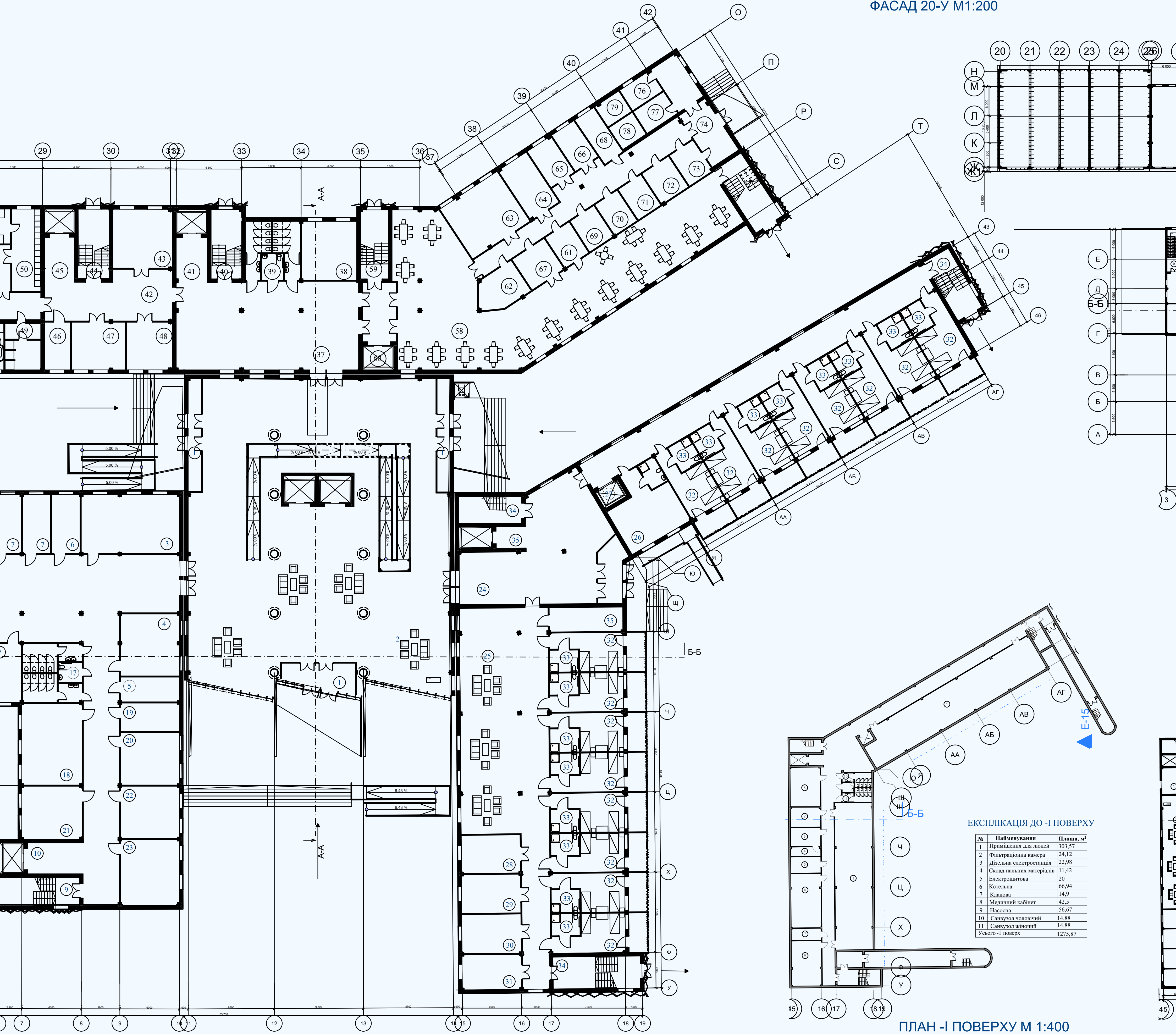
ПЛАН I ПОВЕРХУ
