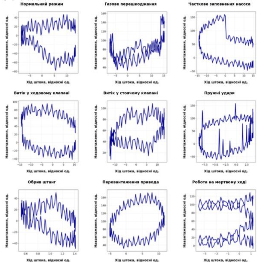
Рисунок 2 - Змодельовані динамограми
