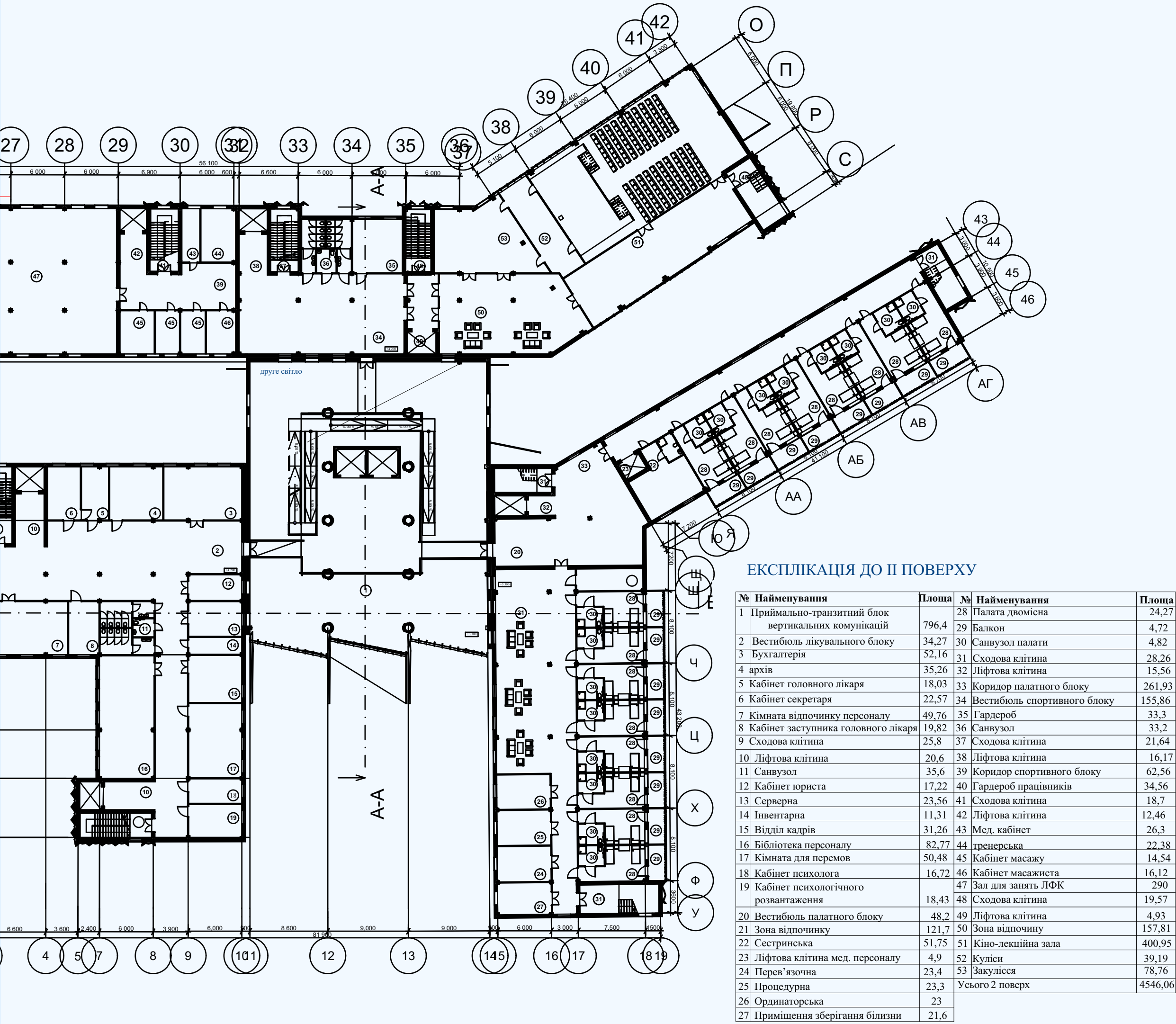
ПЛАН II ПОВЕРХУ М 1:400
