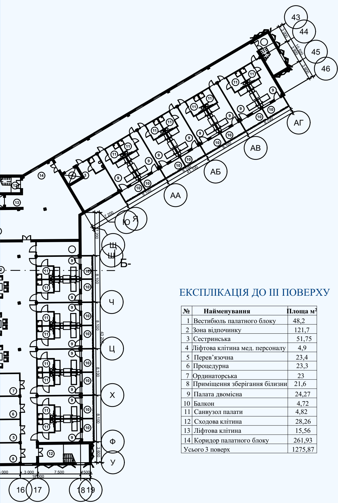
ПЛАН III ПОВЕРХУ М 1:400
