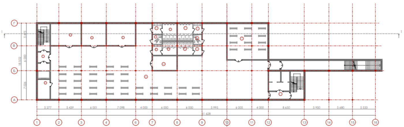
Рисунок 42 – план укриття
