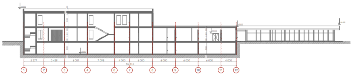
Рисунок 40 – розріз 1-1 м
