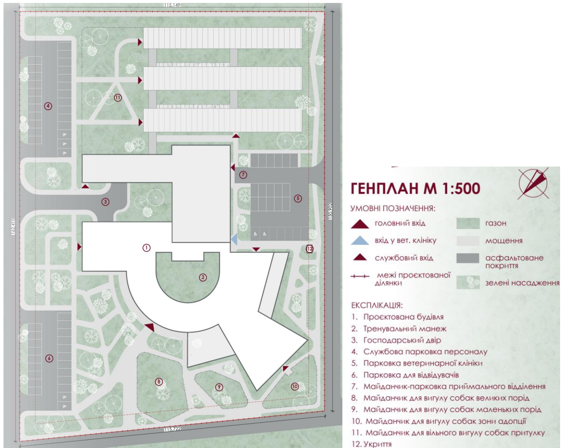
Рисунок 32 – Генеральний план
