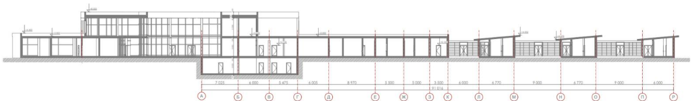
Рисунок 41 – розріз 2-2
