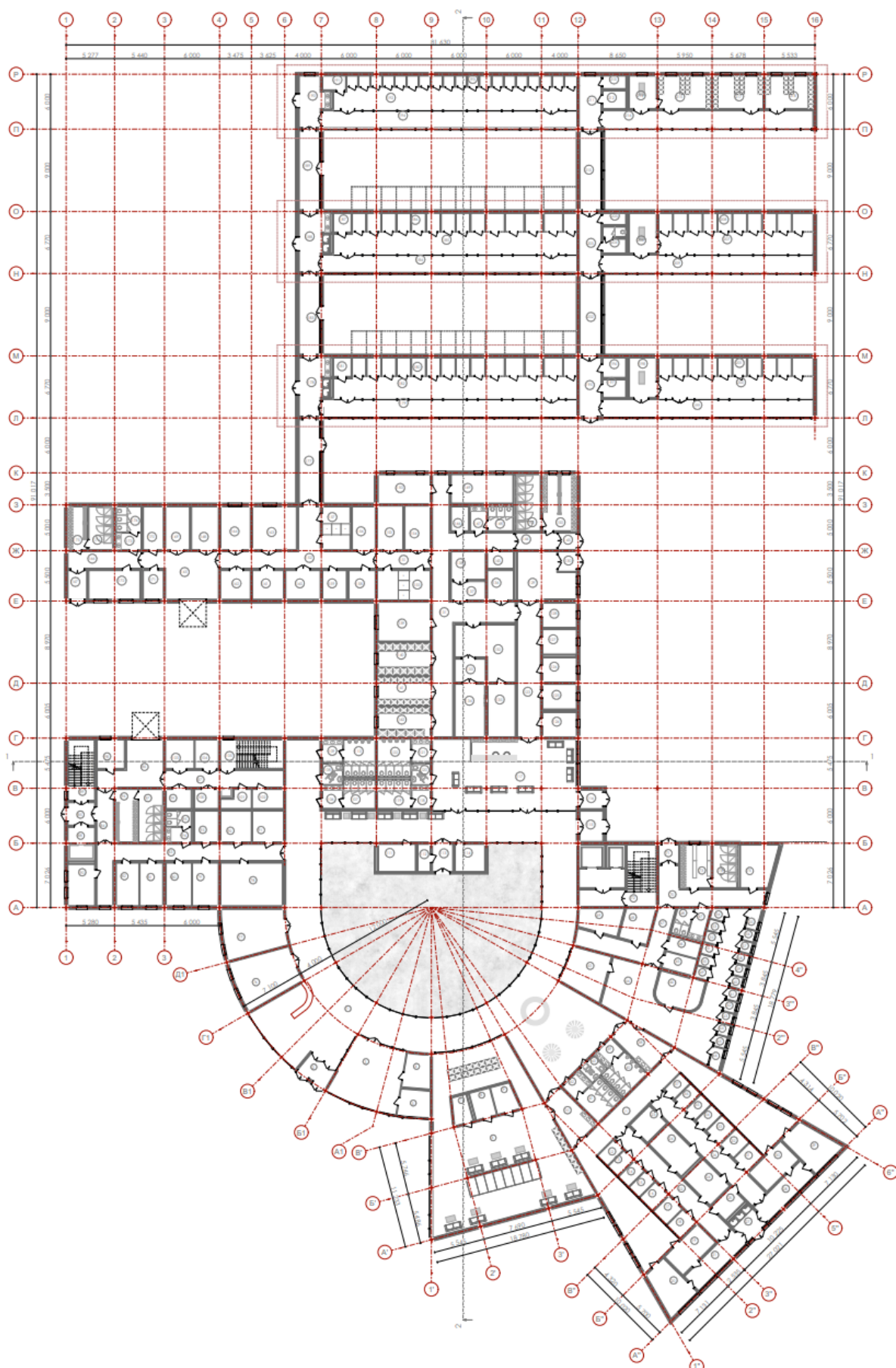
Рисунок 33 – План першого поверху
