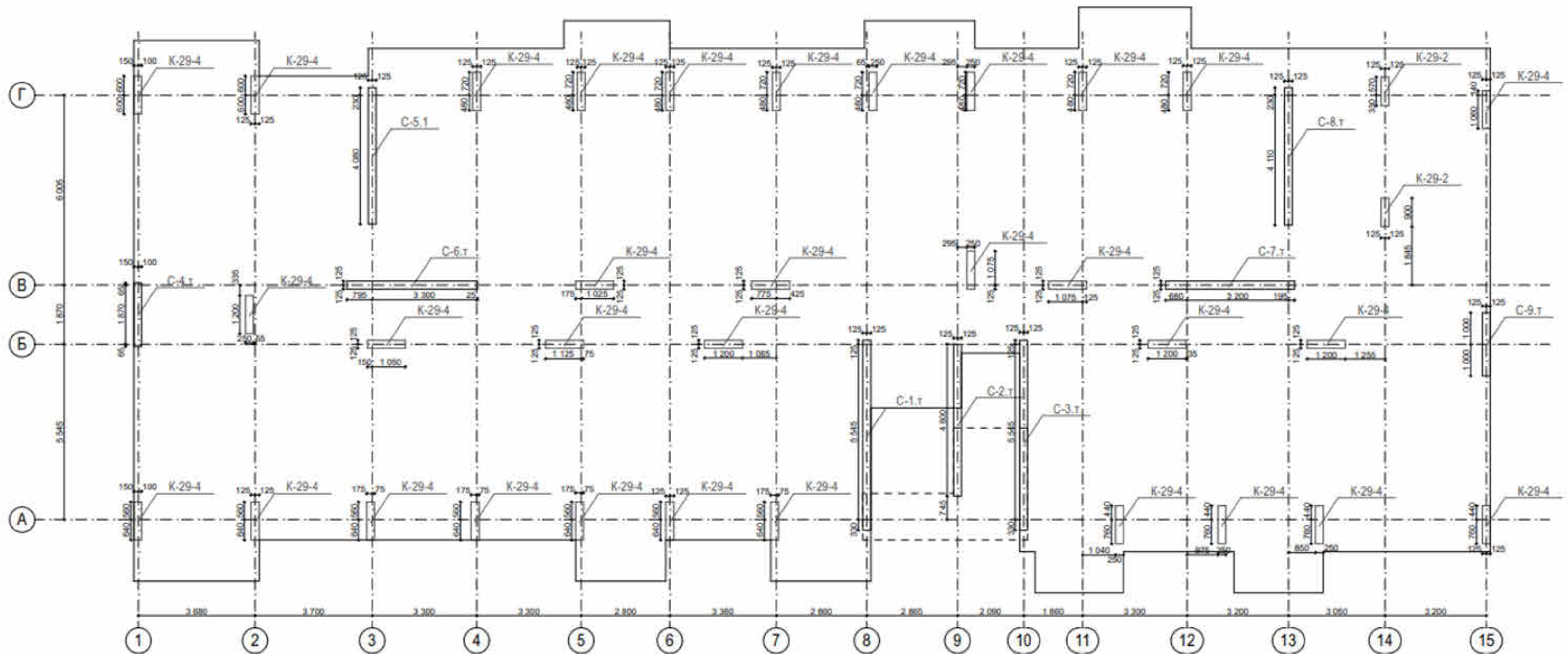
План каркасу типового поверху(2-10 поверх)
