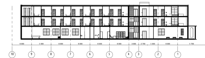
РОЗРІЗ 1-1 М 1:200
