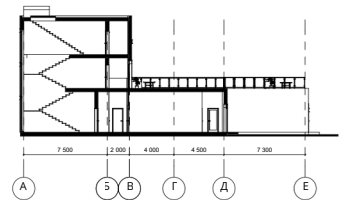
РОЗРІЗ 2-2 М 1:200
