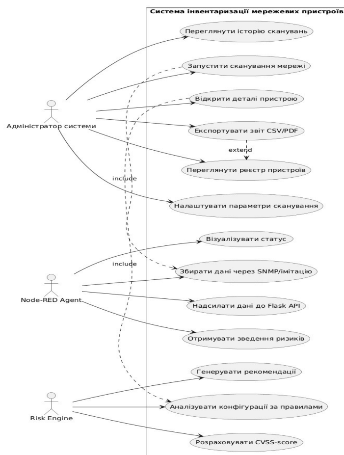
Рисунок 2.3 – Діаграма варіантів використання системи інвентаризації
