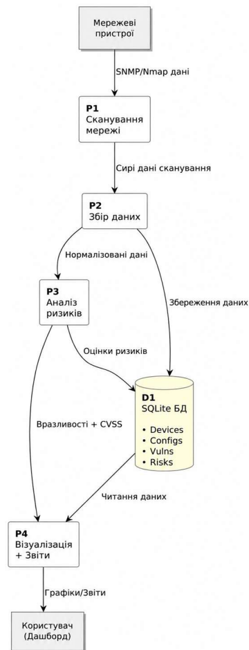
Рисунок 1.5 – DFD Рівень 1: основні процеси обробки даних
