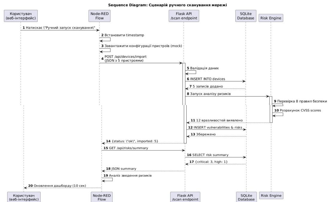
Рисунок 2.4 – Діаграма послідовності сценарію ручного сканування мережі
