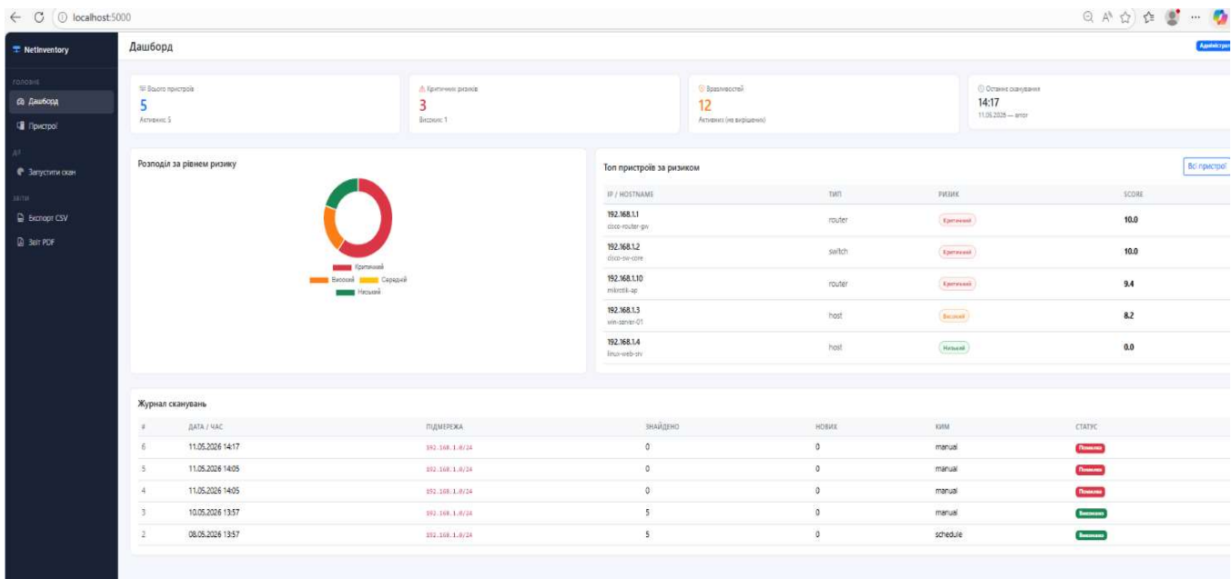
Рисунок 3.7 – Головна сторінка інформаційної панелі (дашборд) вебінтерфейсу системи
