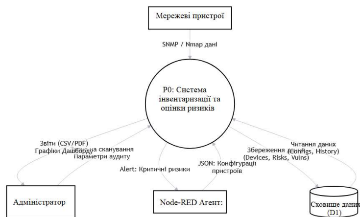
Рисунок 1.4 – DFD Рівень 0 (Контекстна діаграма)
