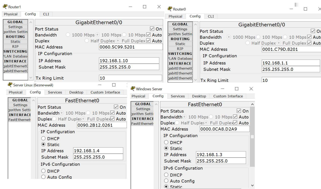
Рисунок 3.12 – Результати конфігурування мережевих пристроїв у середовищі Cisco Packet Tracer
