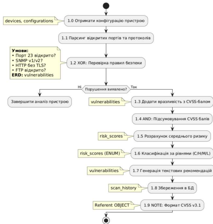
Рисунок 1.6 – Логічна схема потоку робіт аналітичного модуля «Аналіз ризиків»
