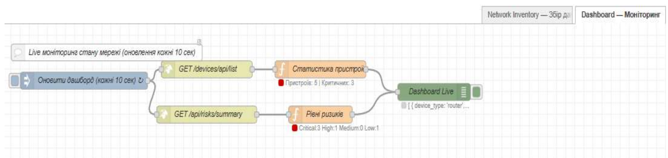
Рисунок 3.5 – Графічна схема підсистеми періодичного оновлення метрик безпеки (вкладка Dashboard — Моніторинг) у середовищі Node-RED
