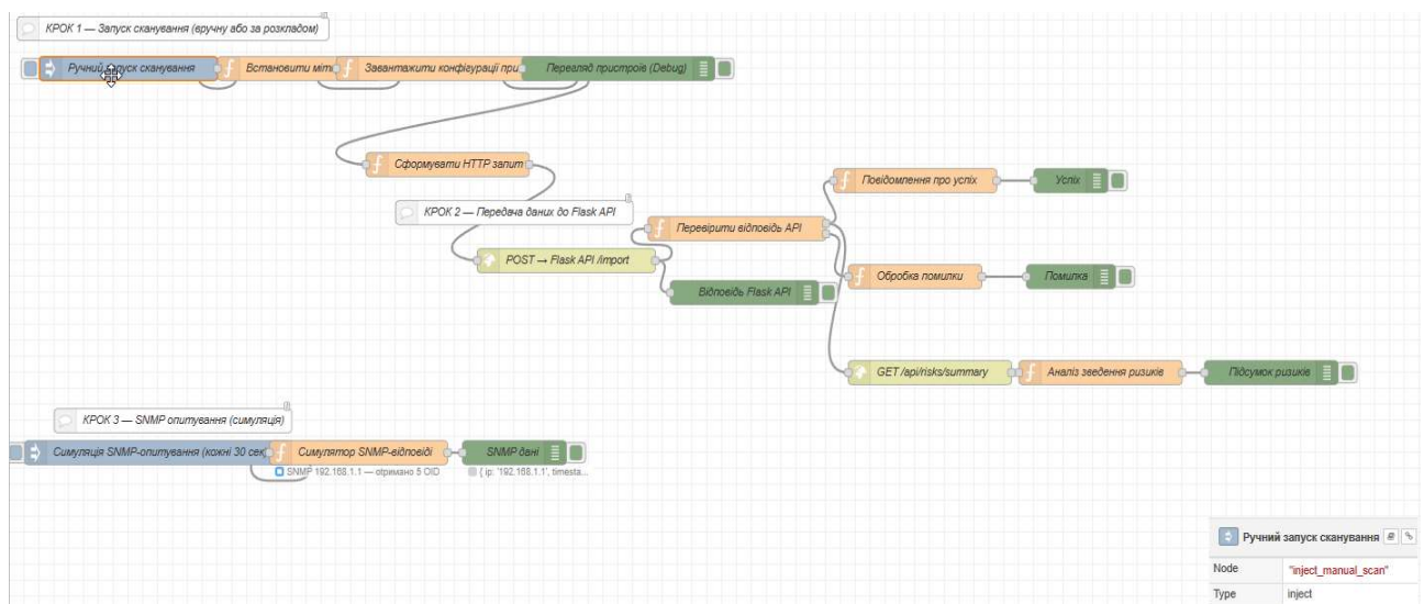
Рисунок 3.3 – Структура потоку інвентаризації та метадані вузла ініціалізації сканування у Node-RED
