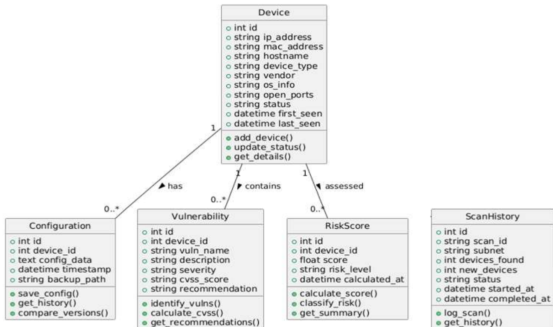
Рисунок 2.1 – Діаграма класів моделі даних системи
