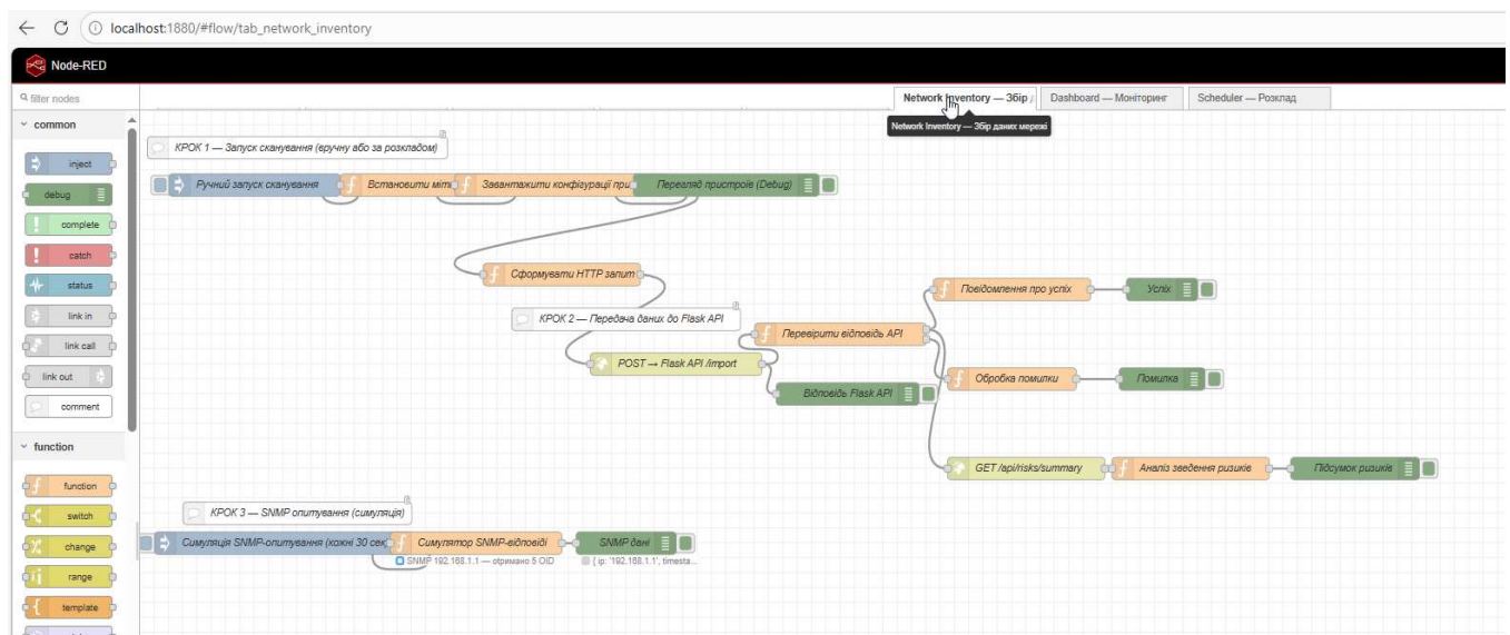
Рисунок 3.2 – Графічна схема потоку збору даних (вкладка Network Inventory) у середовищі Node-RED
