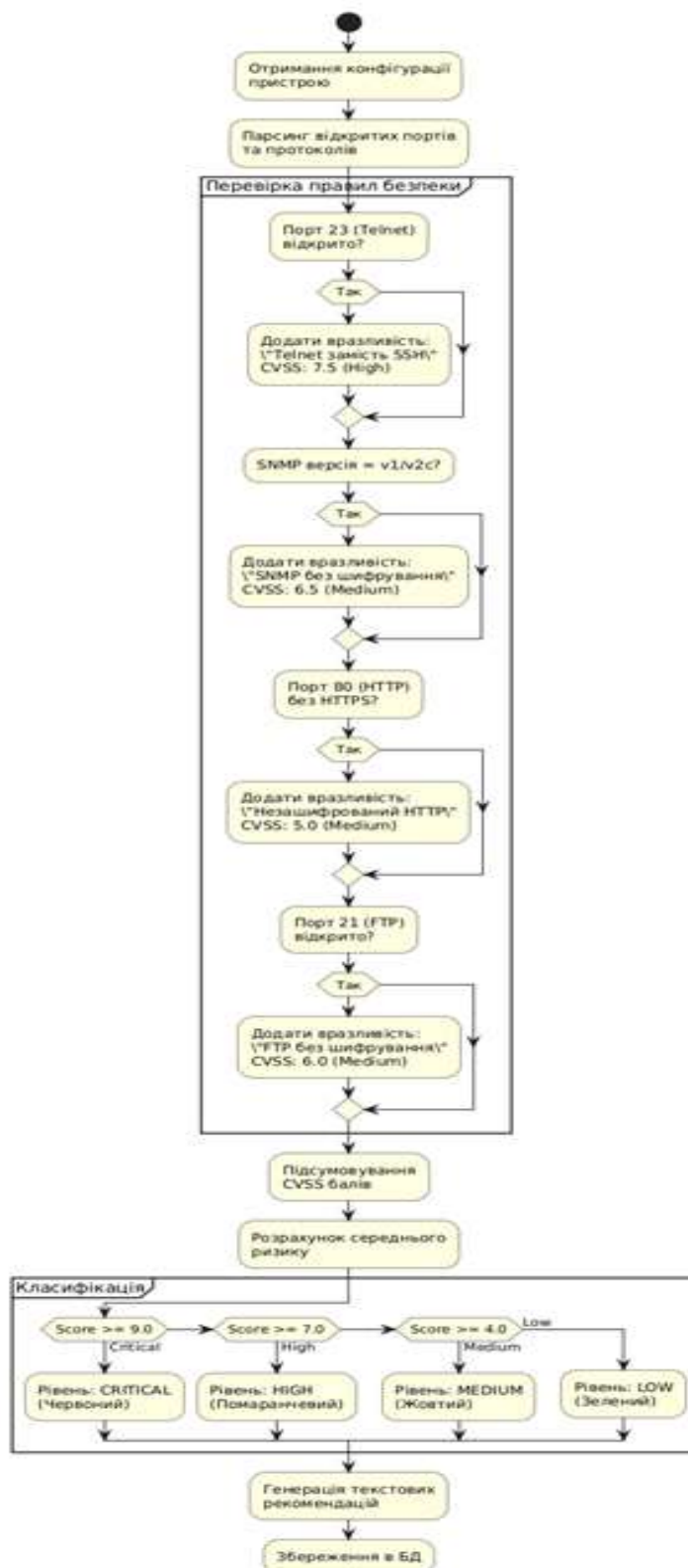
Рисунок 2.2 – Діаграма діяльності алгоритму оцінки ризиків безпеки
