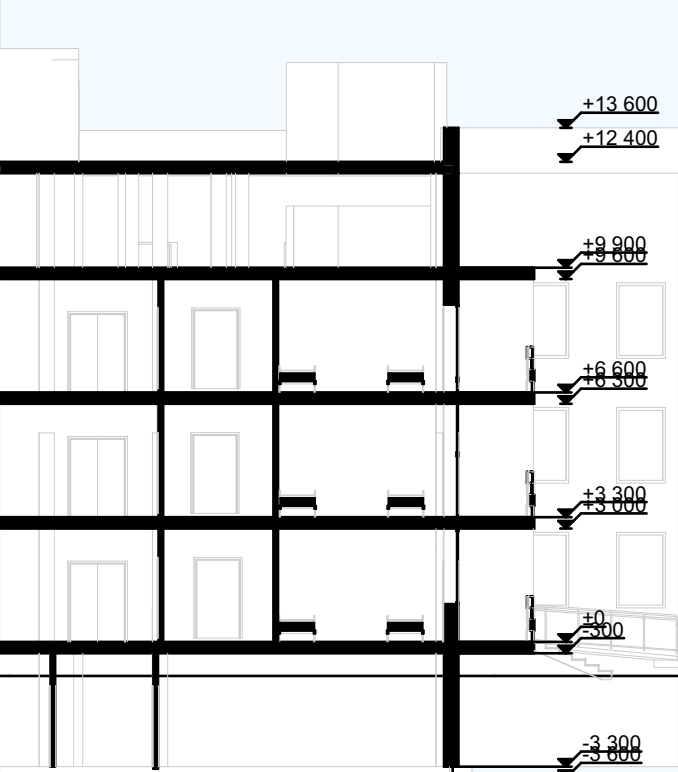
РОЗТИН А-А М1:200
