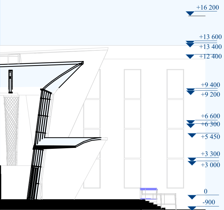
ФАСАД У-О М1:400
