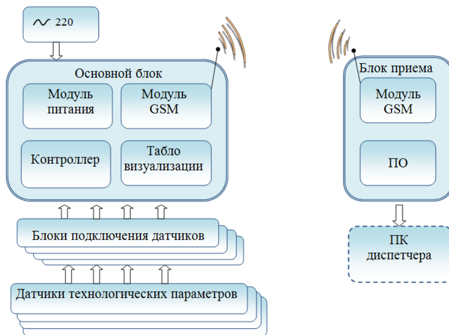
Рисунок 1.22 - Узагальнена структурна схема системи управління ШГНУ з контролем її технічного стану
