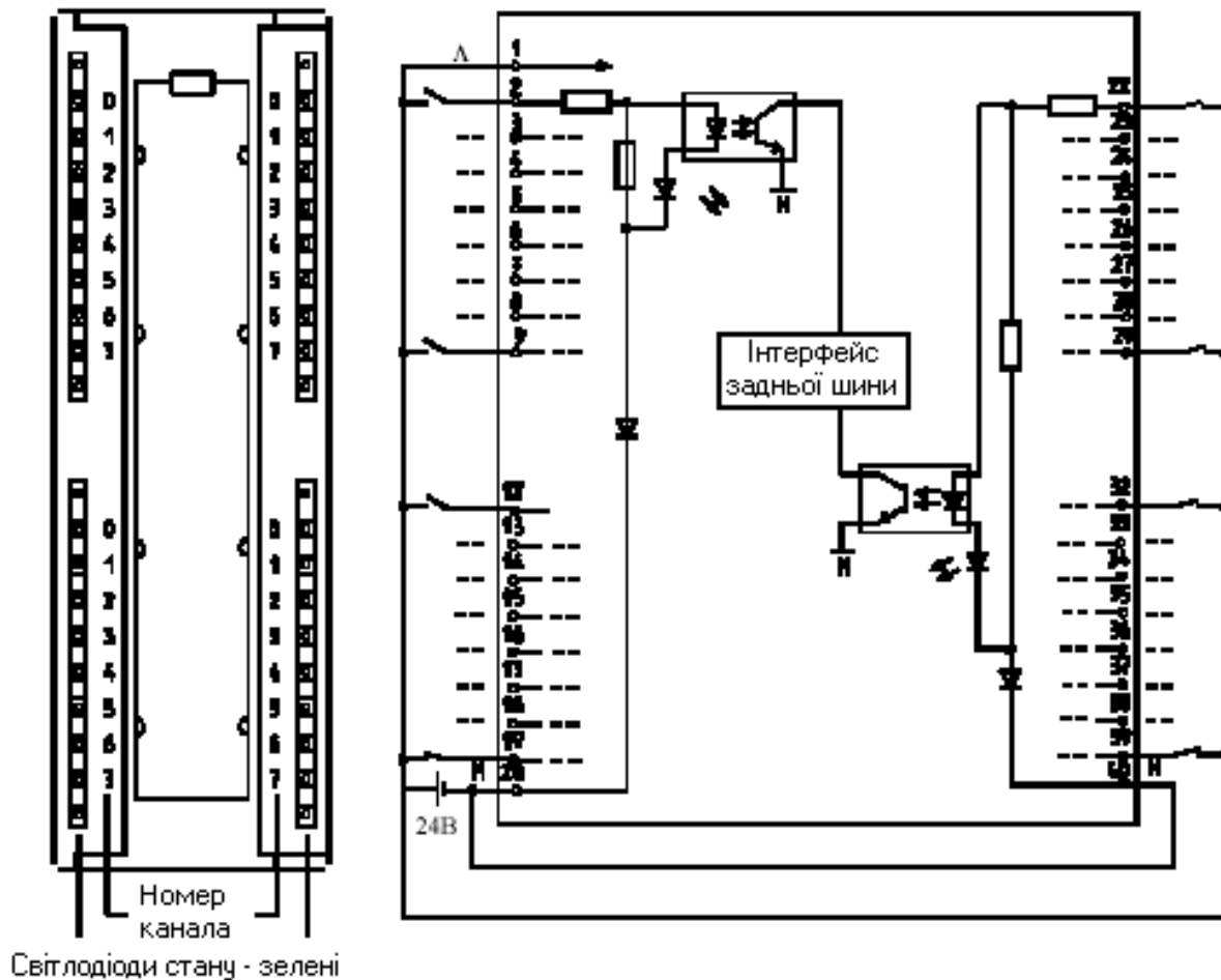
Рисунок 2.16 - Зовнішній вигляд та принципова електрична схема цифрового модуля вводу SM 321; DI 32 x 24 VDC
