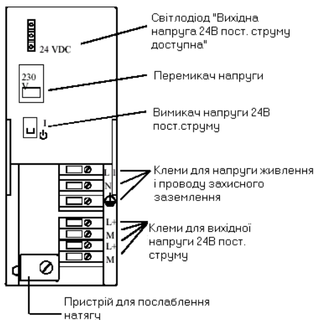
Рисунок 2.12 – Схема електричного підключення блоку живлення PS 307 2A.
