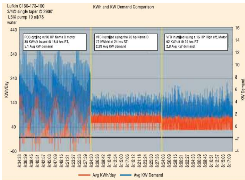
Рисунок 1.17 – Приклад економії потужності при використанні контролера Lufkin Well Manager VSD RPC
