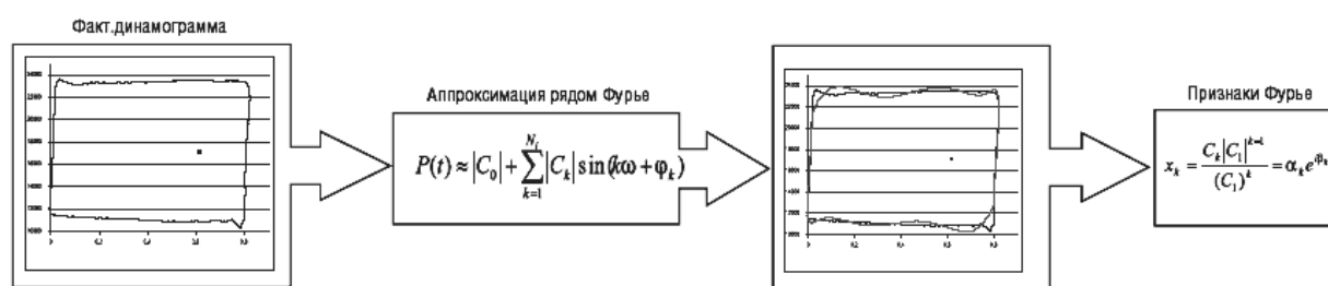
Рисунок 1.8 - Блок-схема алгоритму Алиева – Тер-Хачатурова.
