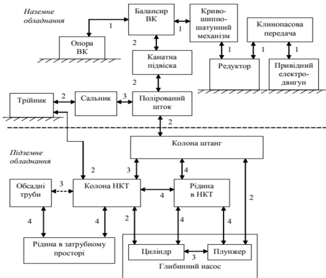
Рис. 1.4 - Структурна схема ШГНУ [4]: 1- жорсткий кінематичний зв'язок; 2 - пружне з'єднання; 3 – сухе і напівсухе тертя; 4 – гідродинамічне тертя.
