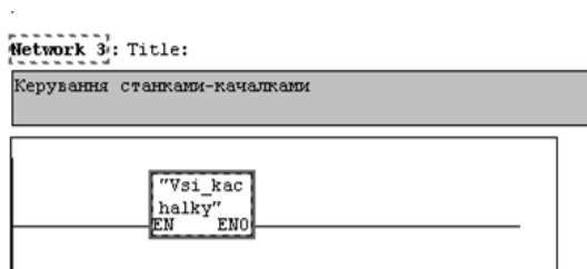
Рисунок 3.5 – Зовнішній вигляд третього Network-а OB1
