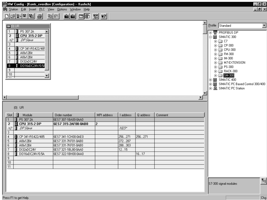
Рисунок 2.11 – Конфігурування комплексу технічних засобів розподіленої системи в Simatic Step7
