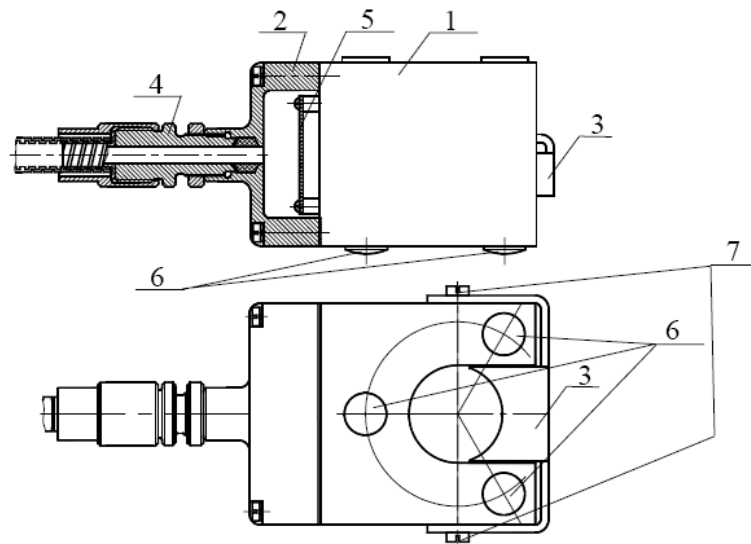
Рисунок 2.6 – Конструктивна схема давача зусилля ДЗ-01
