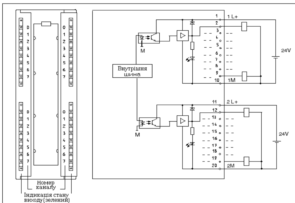
Рисунок 2.14 - Зовнішній вигляд та принципова електрична схема модуля SM 322 (DO 16 x 24 VDC/0.5A)
