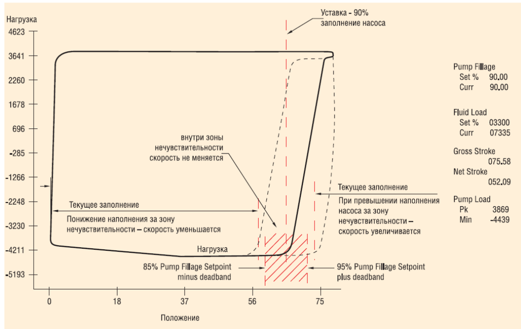
Рисунок 1.15 - Пояснення логіки управління заповненням свердловинного насосу з використанням контролера Lufkin Well Manager VSD RPC
