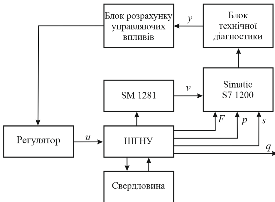
Рисунок 2.3 - Структурна схема системи управління ШГНУ
