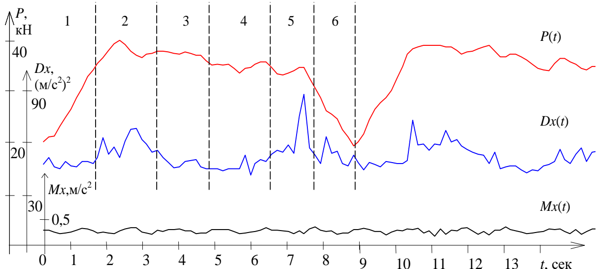
Рисунок 2.2 - Графіки зусилля в штанговій колоні P(t) , зміни математичного очікування Mx(t) і дисперсії Dx(t) вібраційного процесу в часі
