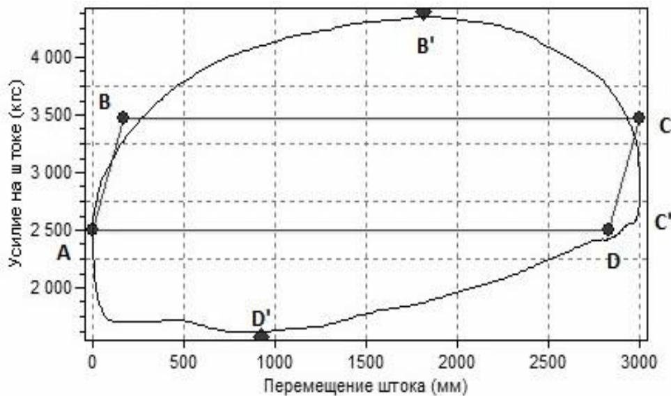
Рисунок 1.11 - Практична динамограма роботи насоса під час витoku рідини в нагнітальному вузлі
