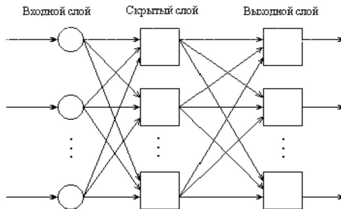
Рисунок 1.6 - Структура нейронної двошарової прямоспрямованої мережі для аналізу динамограм [8]
