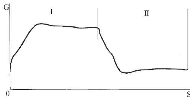
Рисунок 2.1 - Типова розгорнута динамограма
