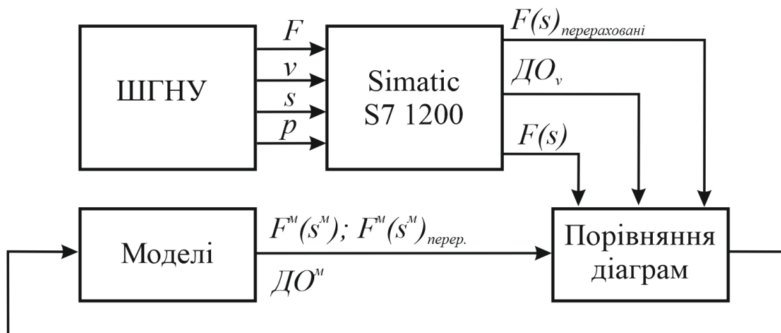
Рисунок 2.4 - Структурна схема блоку технічної діагностики ШГНУ
