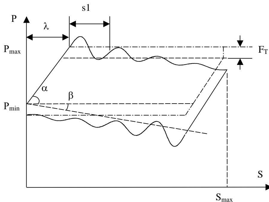
Рисунок 1.3 – Динамограма нормальної роботи ШГНУ [4]
