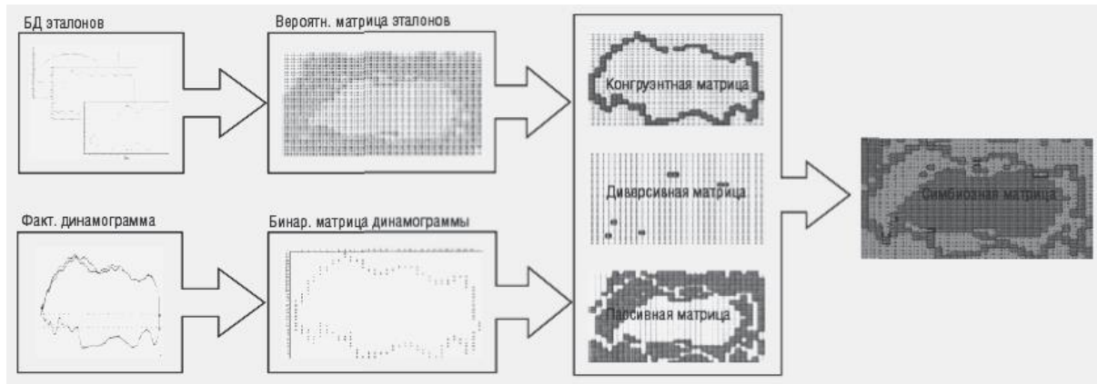
Рисунок 1.7 - Блок-схема алгоритму Оганезова [8]
