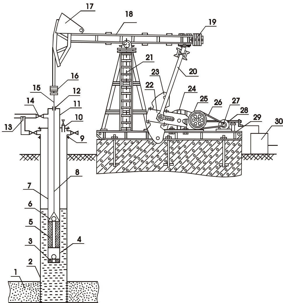
Рисунок 1.1 – Загальна конструктивна схема штангової глибинно-насосної установки [1].
