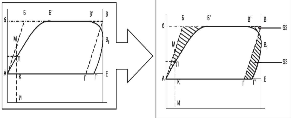
Рисунок 1.10 - Діагностика витoku рідини в нагнітальній частині насоса.
