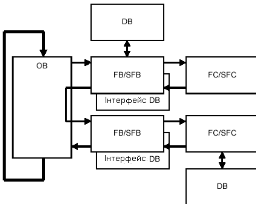
Рисунок 3.1 – Порядок виклику блоків
