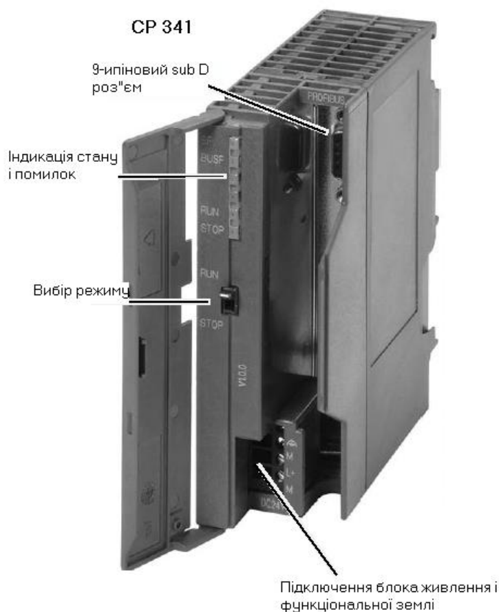
Рисунок 2.13 – Зовнішній вигляд комунікаційного процесора CP 341
