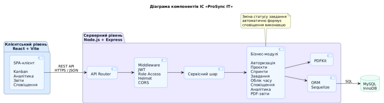
Рисунок 2.8 — Діаграма компонентів системи «ProSync IT»
