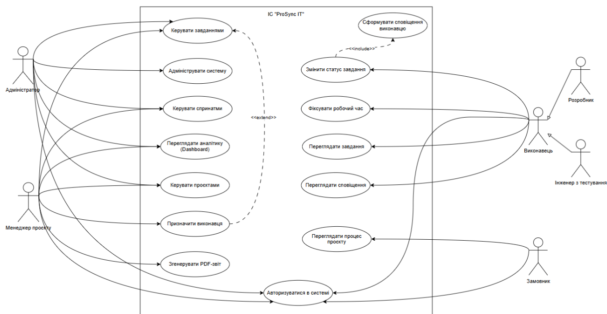
Рисунок 1.4 — Діаграма прецедентів (Use Case) IC «ProSync IT»
