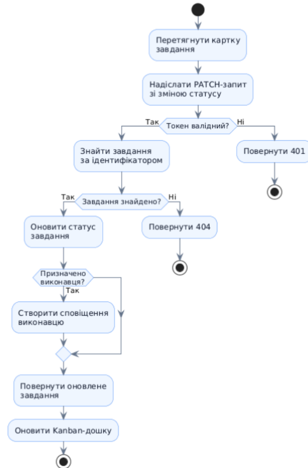
Рисунок 2.12 — Діаграма діяльності процесу зміни статусу завдання
