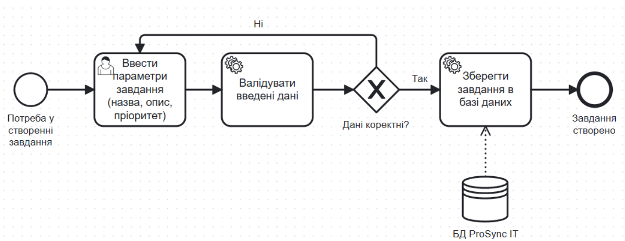
Рисунок 2.5 — Діаграма бізнес-процесу створення завдання в беклозі
