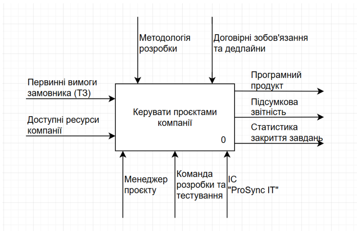
Рисунок 2.1 — Контекстна діаграма IDEF0 (A-0)
