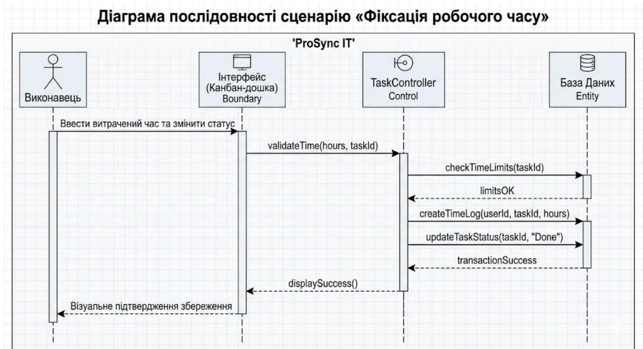
Рисунок 2.11 — Діаграма послідовності сценарію «Зміна статусу завдання»
