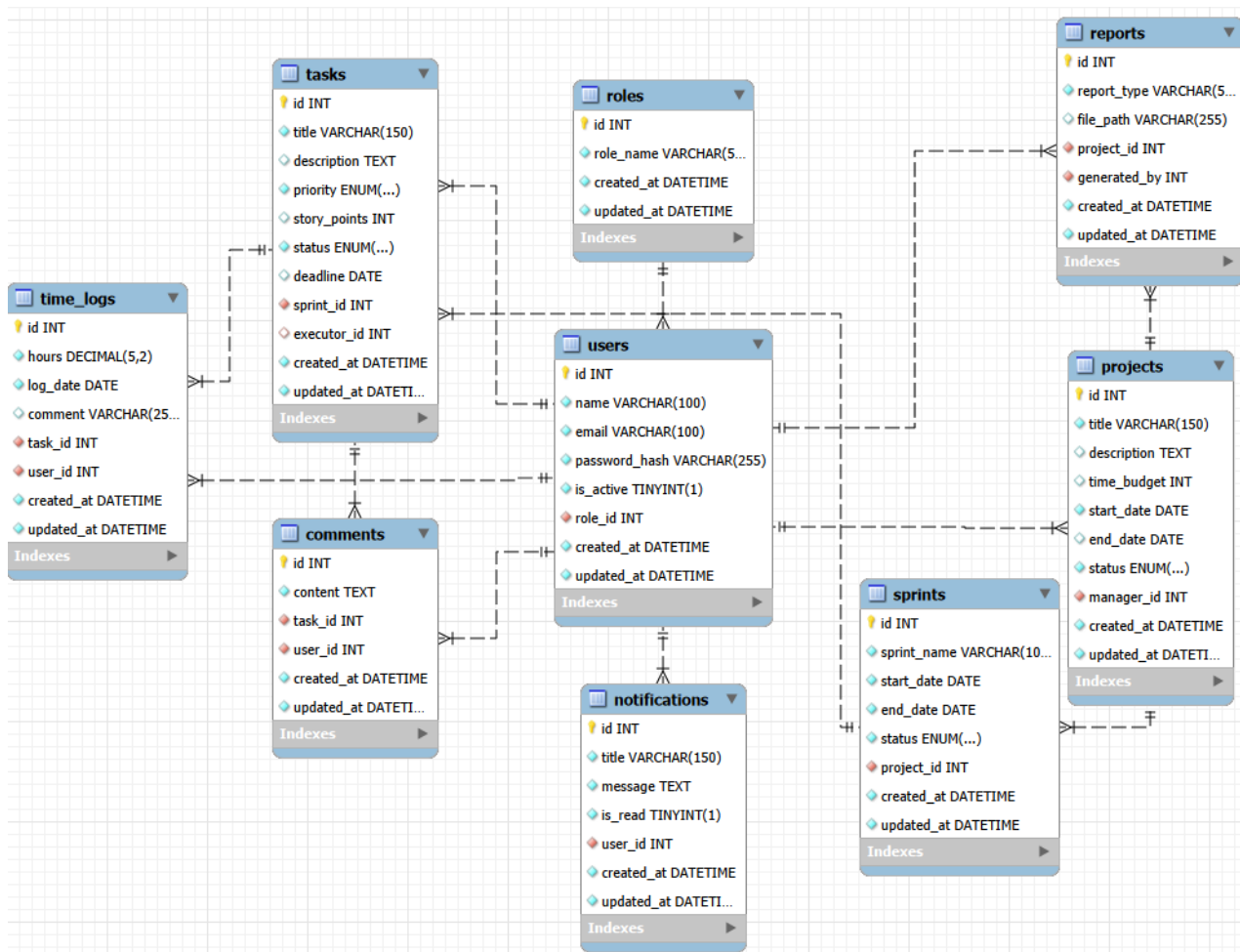
Рисунок 2.13 — Концептуальна ER-діаграма бази даних «ProSync IT»
