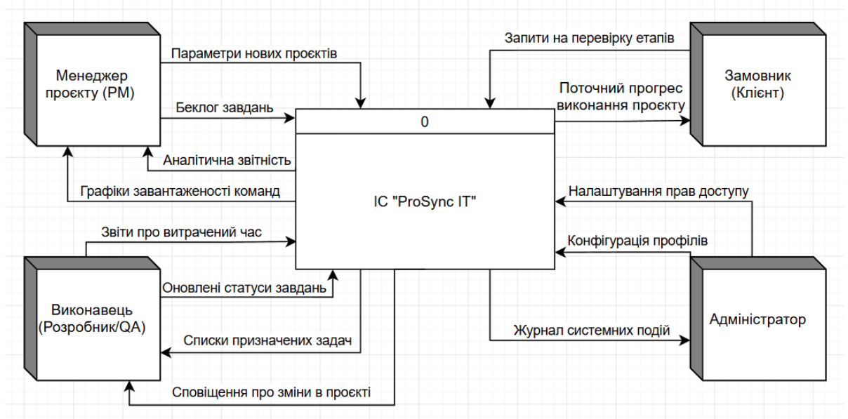
Рисунок 2.3 — Контекстна діаграма потоків даних (DFD)
