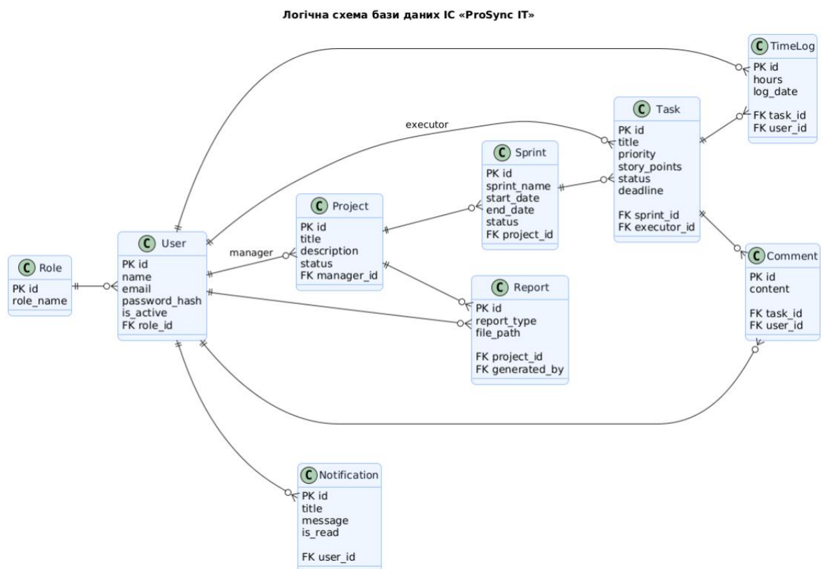
Рисунок 2.14 — Логічна схема реляційної бази даних «ProSync IT»
