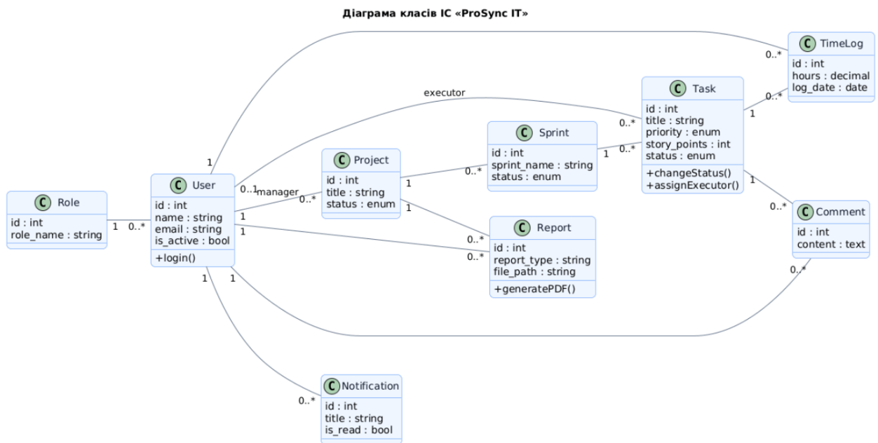
Рисунок 2.10 — Діаграма класів системи «ProSync IT»
