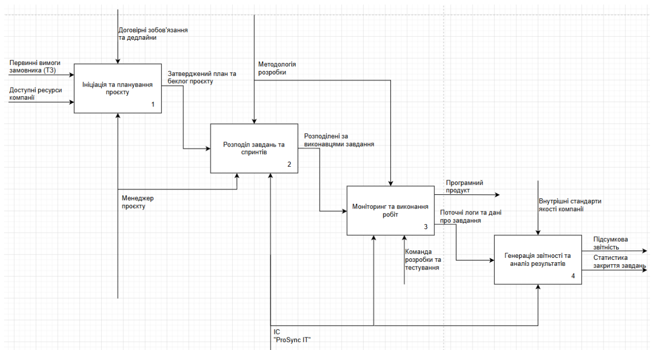
Рисунок 2.2 — Діаграма декомпозиції IDEF0 (A0)
