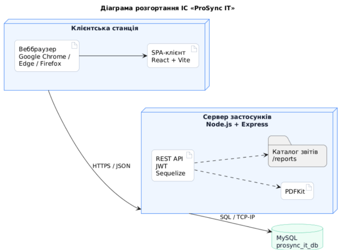
Рисунок 2.9 — Діаграма розгортання системи «ProSync IT»
