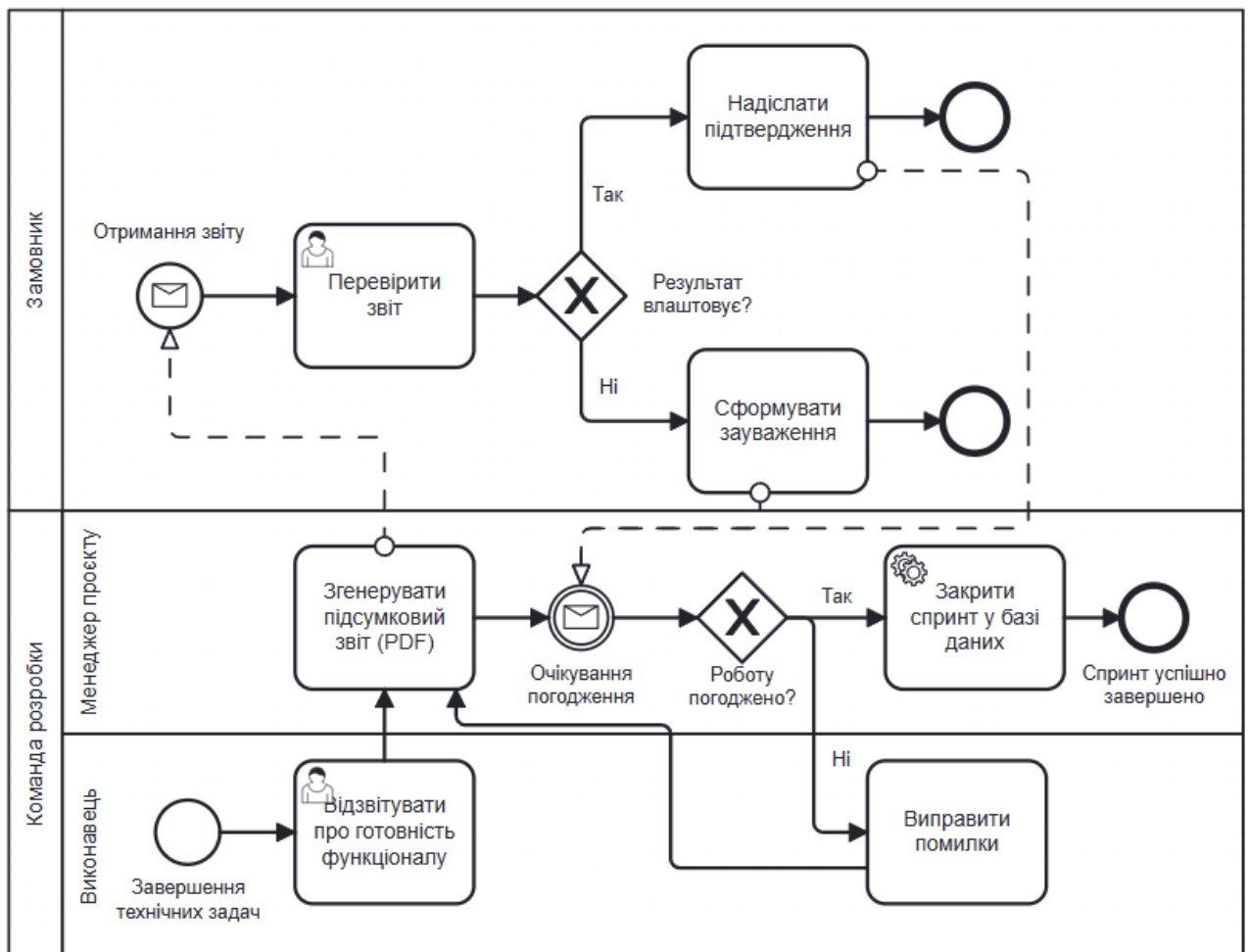
Рисунок 2.7 — Діаграма бізнес-процесу погодження результатів спринту
