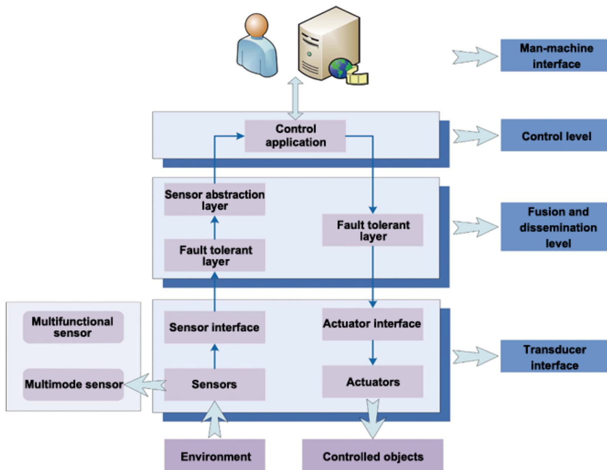
Рис. 1.1 — Структура інтелектуальної мультисенсорної системи.
