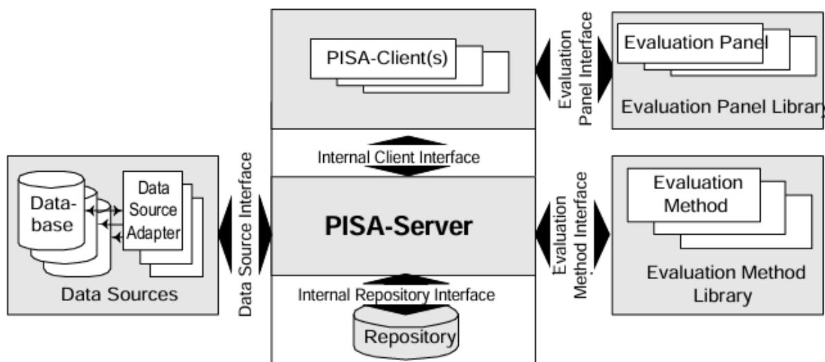
Рис. 2.6 - Архітектура
