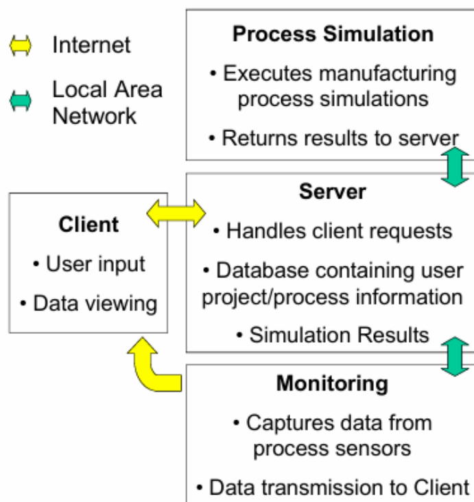
Рис. 2.1 - Схема системи
