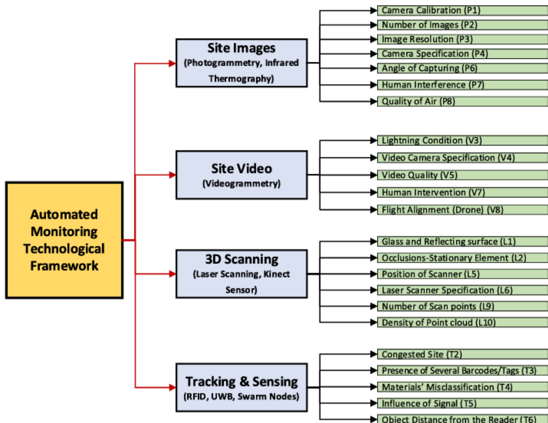
Рис. 3.6 - Модель автоматизованого моніторингу на основі технологій.
