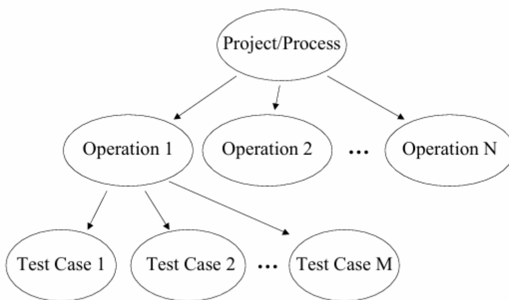
Рис. 2.2 - Структура проекту
