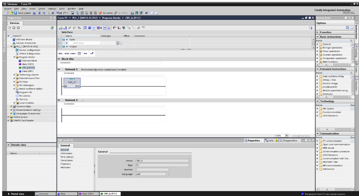
Рисунок 2.18 – Вікно додавання функції FC1
