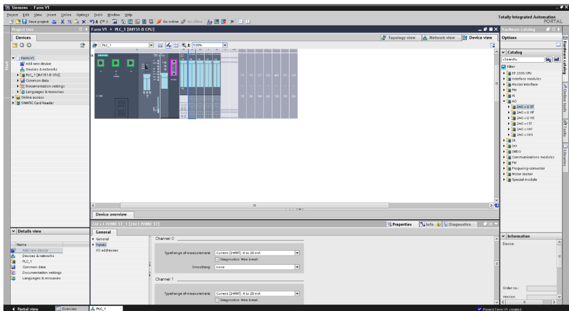
Рисунок 2.9 – Параметрування аналогового вводу 2AIx12WIRE ST
