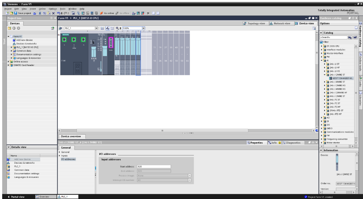
Рисунок 2.8 – Модулі аналогового вводу 2AIx12WIRE ST
