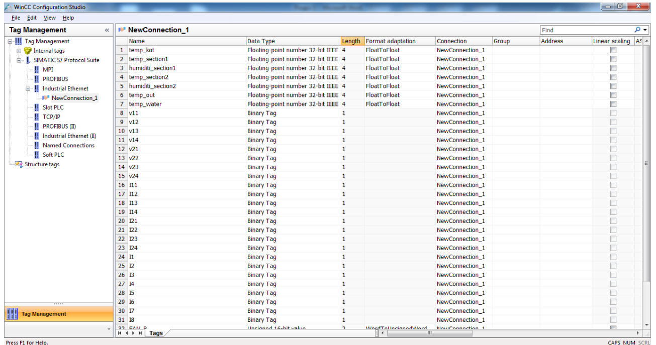
Рисунок 3.12 – Теги проекту
