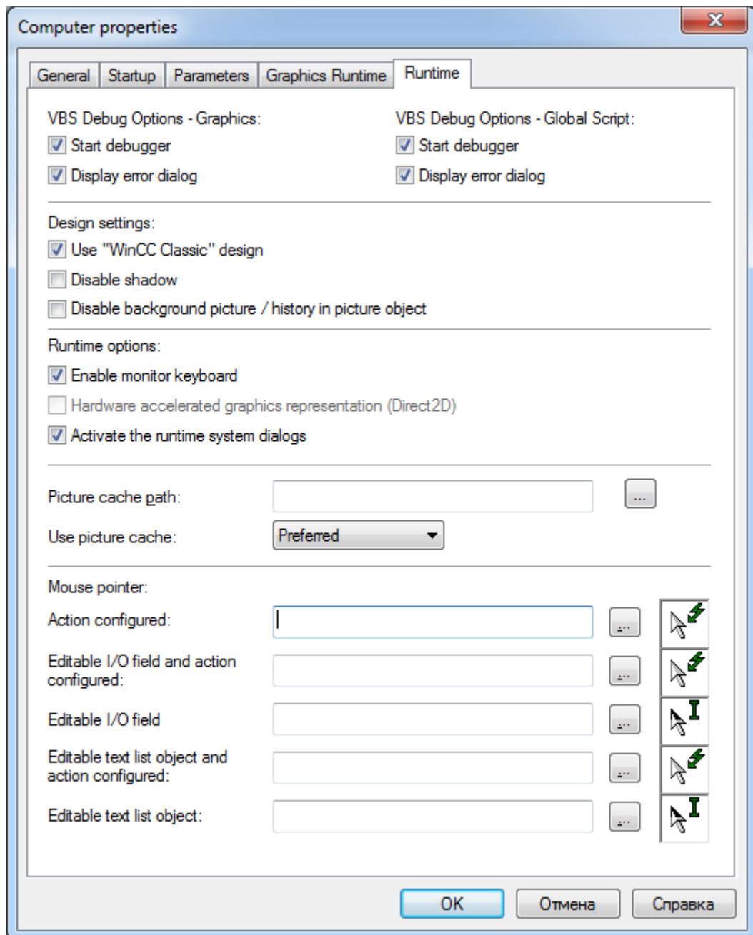
Рисунок 3.7 – Вікно налаштування запуску проекту
