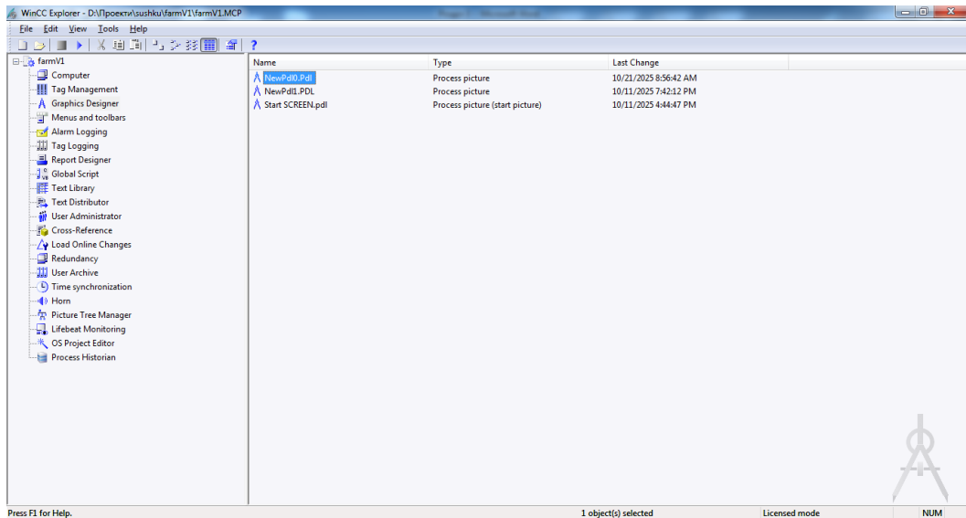
Рисунок 3.13 – Вікна проекту
