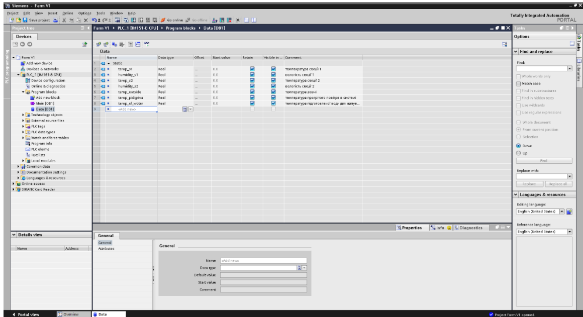
Рисунок 2.16 – Блок даних та теги для збереження значень температури та вологості
