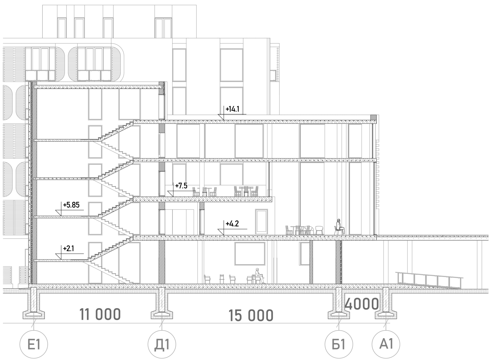
РОЗРІЗ Н-Н М 1:200
