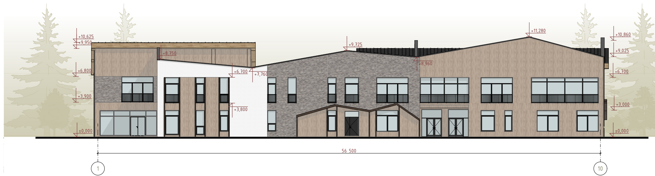
ФАСАД 1-10 М 1:250
