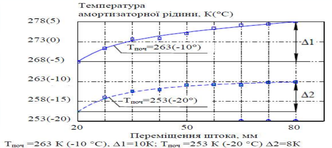
Рисунок 13.2 – Залежність температури амортизаторної рідини від переміщення штока гідравлічних амортизаторів КрА3-260
