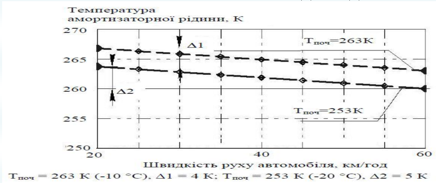
Рисунок 12.1 – Залежність усталеної температури амортизаторної рідини від швидкості руху установки для капітального ремонту свердловин АОРС-60 на шасі КрАЗ-260
