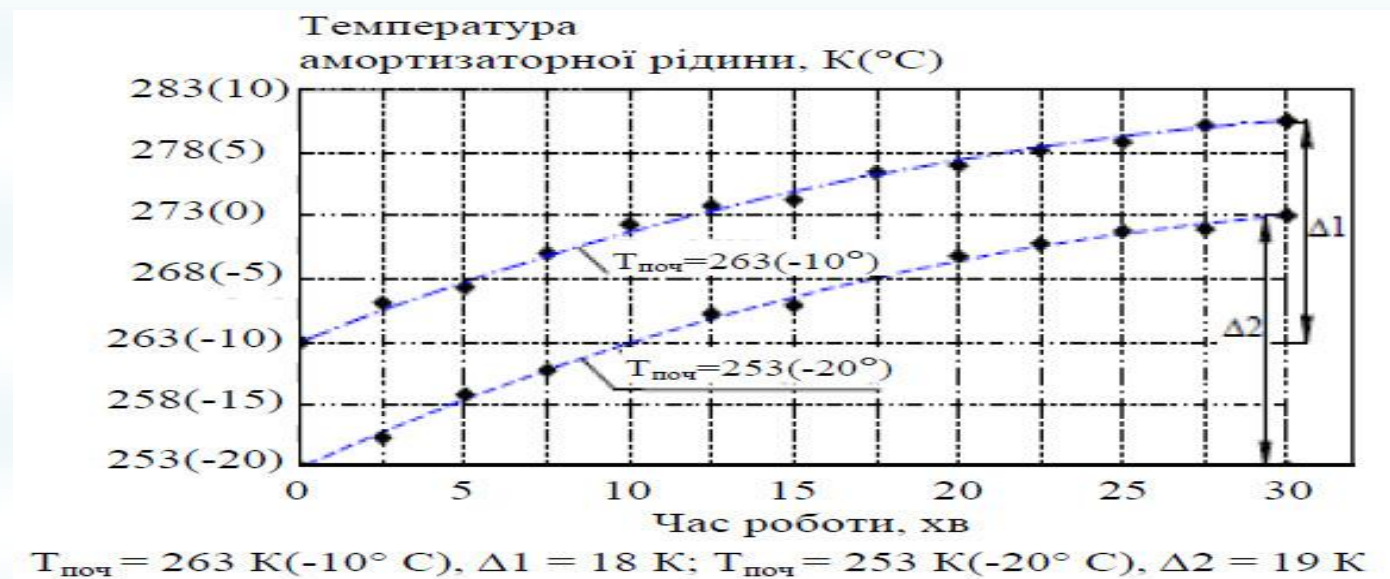
Рисунок 12.2 – Залежність усталеної температури амортизаторної рідини від часу роботи амортизатора установки для капітального ремонту свердловин АОРС-60 на шасі КрАЗ-260
