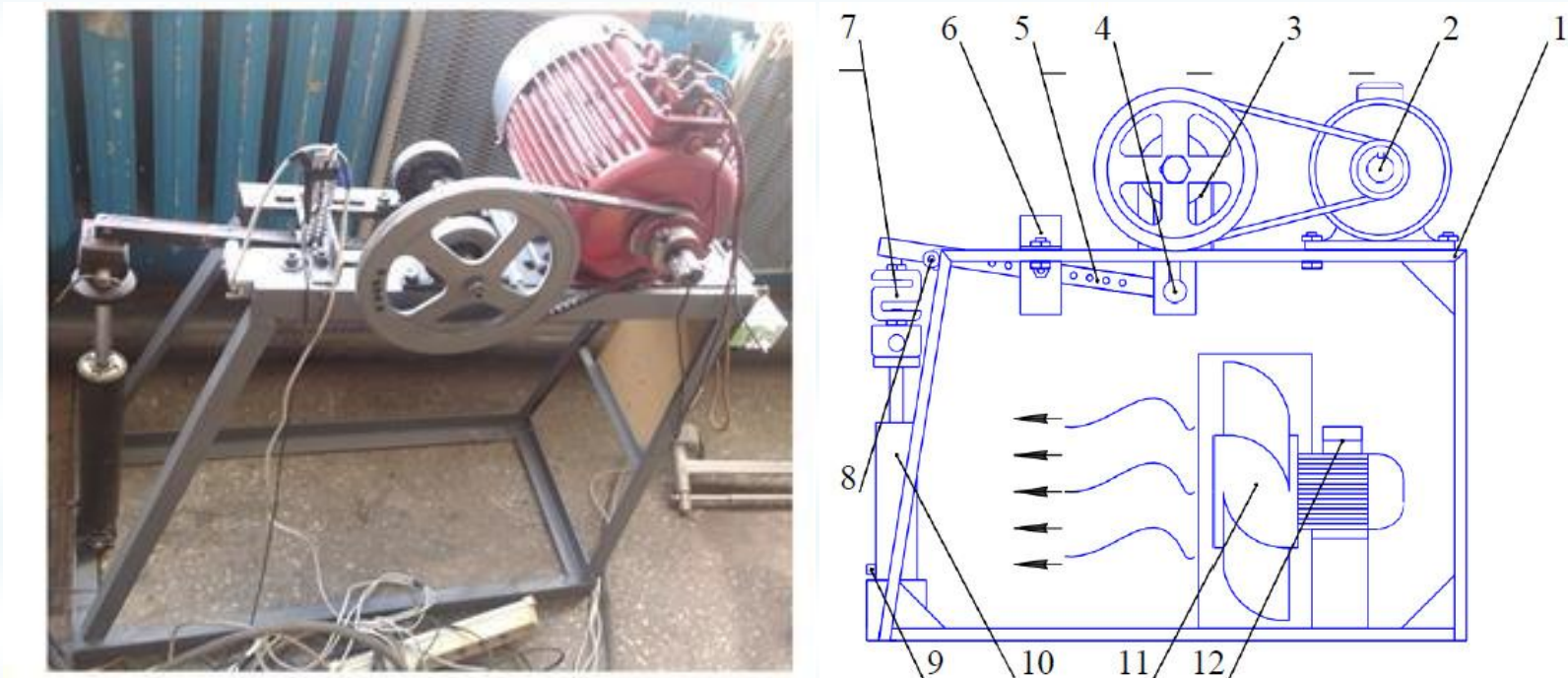
Рисунок 11 – Промислова експериментальна установка для визначення експлуатаційних характеристик амортизаторів
