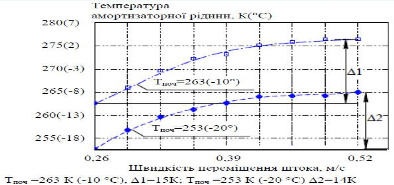
Рисунок 13.1 – Залежність усталеної температури амортизаторної рідини від швидкості переміщення штока
