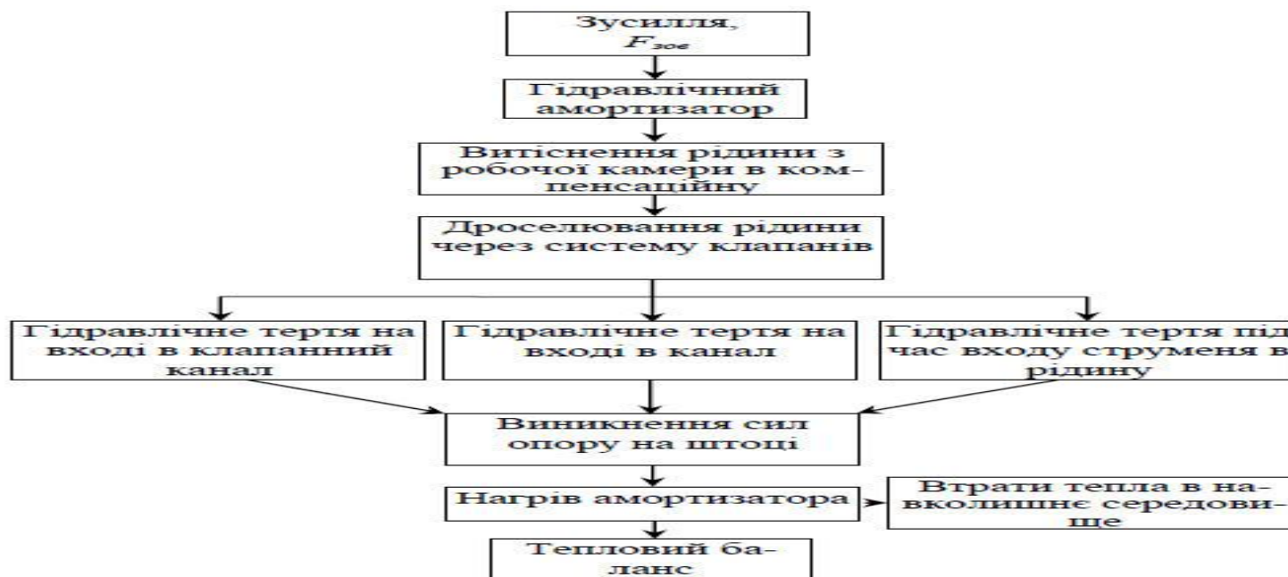
Рисунок 4.2 – Взаємозв'язок процесів, що виникають у результаті перетворення механічної енергії в теплову під час роботи гідравлічного амортизатора
