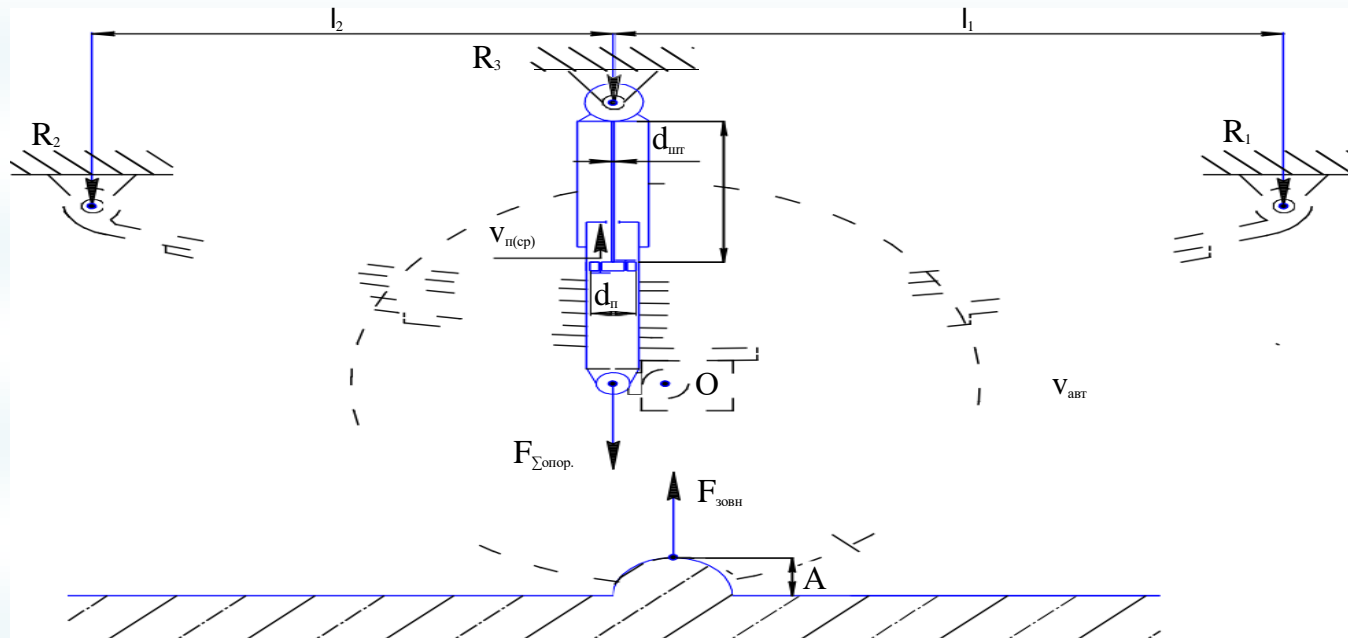
Рисунок 5.2 – Схема сил в амортизаторі, діючих в результаті наїзду колеса на перешкоду
