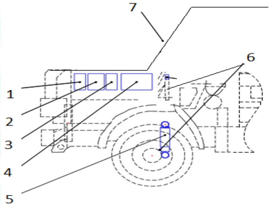
Рисунок 10.1 – Експериментальна установка АОРС-60 на базі автомобіля КрАЗ-260 із встановленими датчиками контролю температури амортизаторної рідини і температури навколишнього повітря
