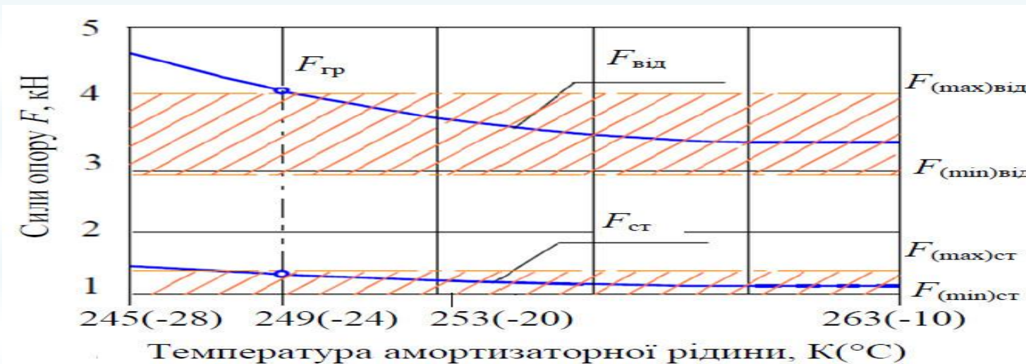
Рисунок 7.2 – Теоретична залежність зміни сил опору гідравлічного амортизатора від температури експлуатації
