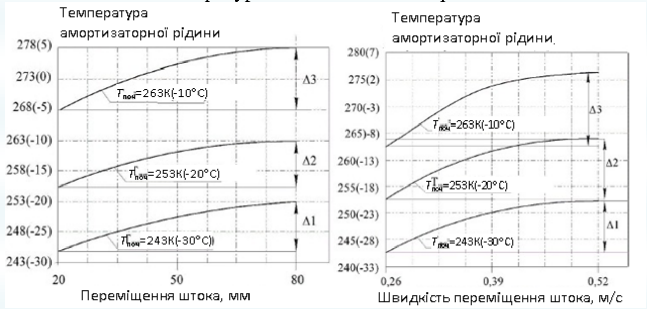
Рисунок 8.2 – Залежність усталеної температури амортизатора від величини та швидкості переміщення штока
