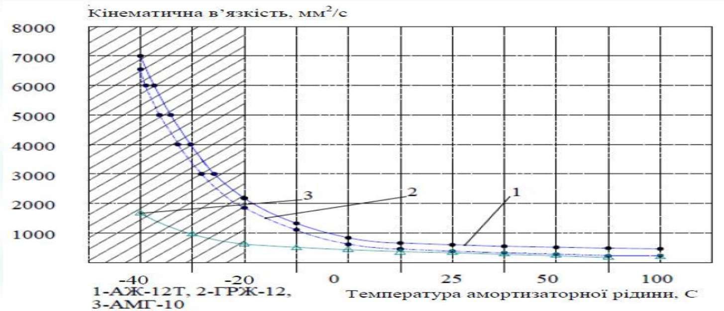
Рисунок 7.1 – Залежність зміни кінематичної в'язкості амортизаторної рідини різних марок від її температури
