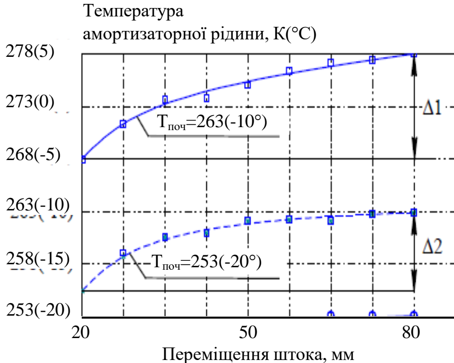
Рисунок 4.4 – Залежність температури амортизаторної рідини від переміщення штока гідравлічних амортизаторів КрАЗ-260
