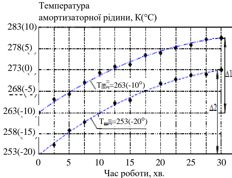
Рисунок 4.2 – Залежність усталеної температури амортизаторної рідини від часу роботи амортизатора установки для капітального ремонту свердловин АОРС-60 на шасі КраЗ-260
