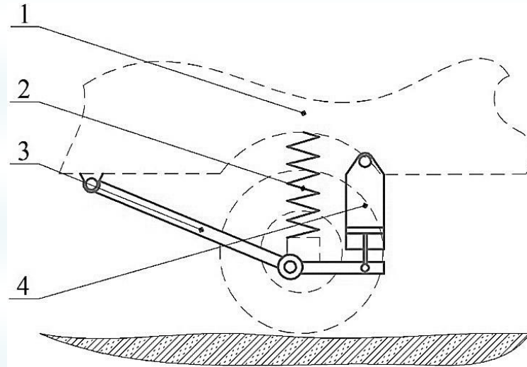
1 - опорна частина кузова; 2 - пружний елемент; 3 – напрямний пристрій; 4 - амортизатор Рисунок 5.1 – Схема взаємодії елементів підвіски автомобілів
