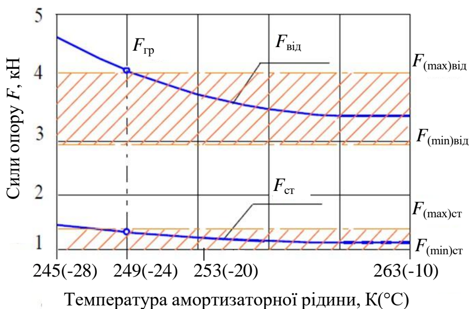
Рисунок 2.3 – Теоретична залежність зміни сил опору гідравлічного амортизатора від температури експлуатації
