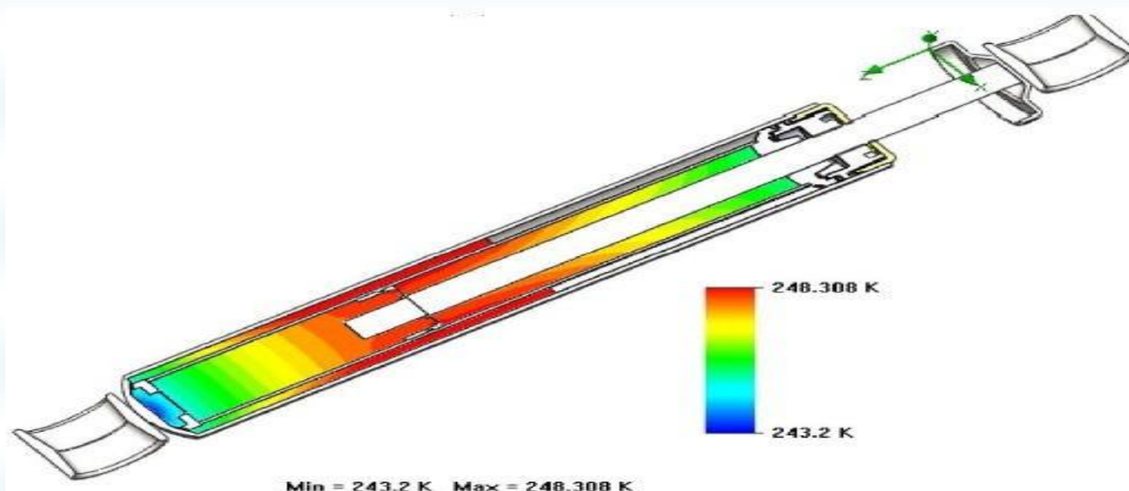
Рисунок 9.2 – Графічне зображення моделювання температури амортизатора вантажного автомобіля КрАЗ
