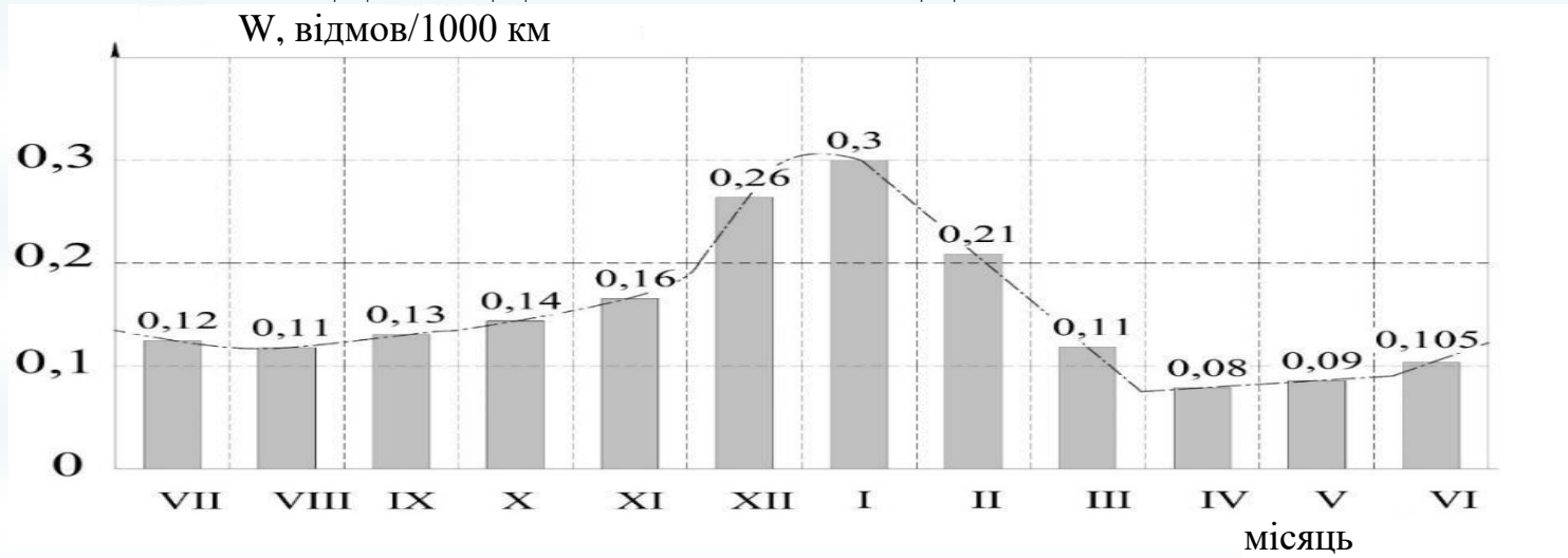
Рисунок 2.1 – Розподіл відмов вузлів підвіски автомобілів по місяцям року
