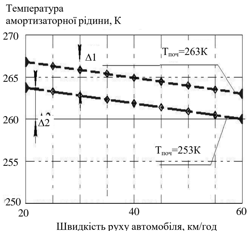
Рисунок 4.1 – Залежність усталеної температури амортизаторної рідини від швидкості руху автомобіля
