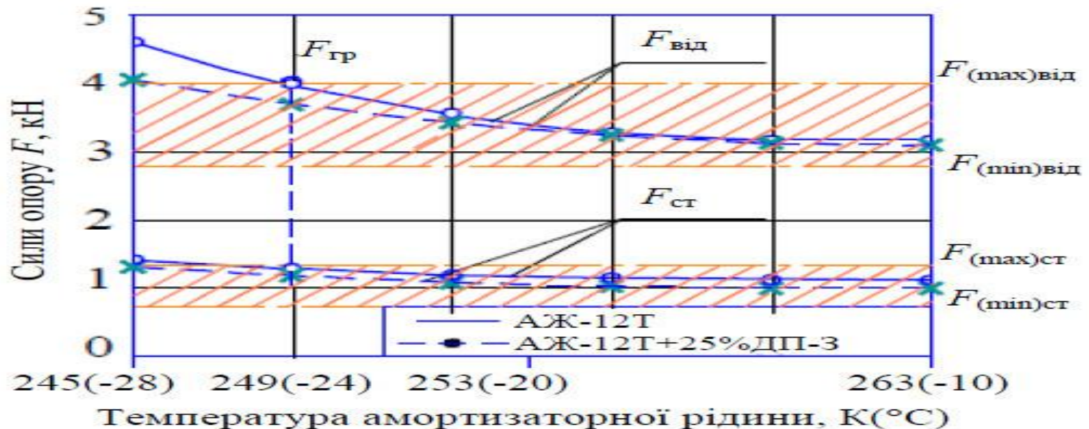
Рисунок 14.2 – Залежність зміни сил опору на відбій ( F_{відб} ) та стиск ( F_{см} ) у випадку використання амортизаторної рідини АЖ-12Т і модифікованої за низьких температур експлуатації
