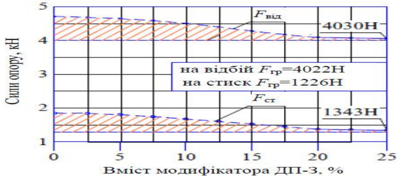
Рисунок 14.1 – Залежності зміни сил опору на відбій ( F_{відб} ) та стиск ( F_{см} ) гідравлічних амортизаторів із вмістом модифікатора ДП-3 у загальному об'ємі амортизаторної рідини для температури експлуатації 259К (-14 °С)
