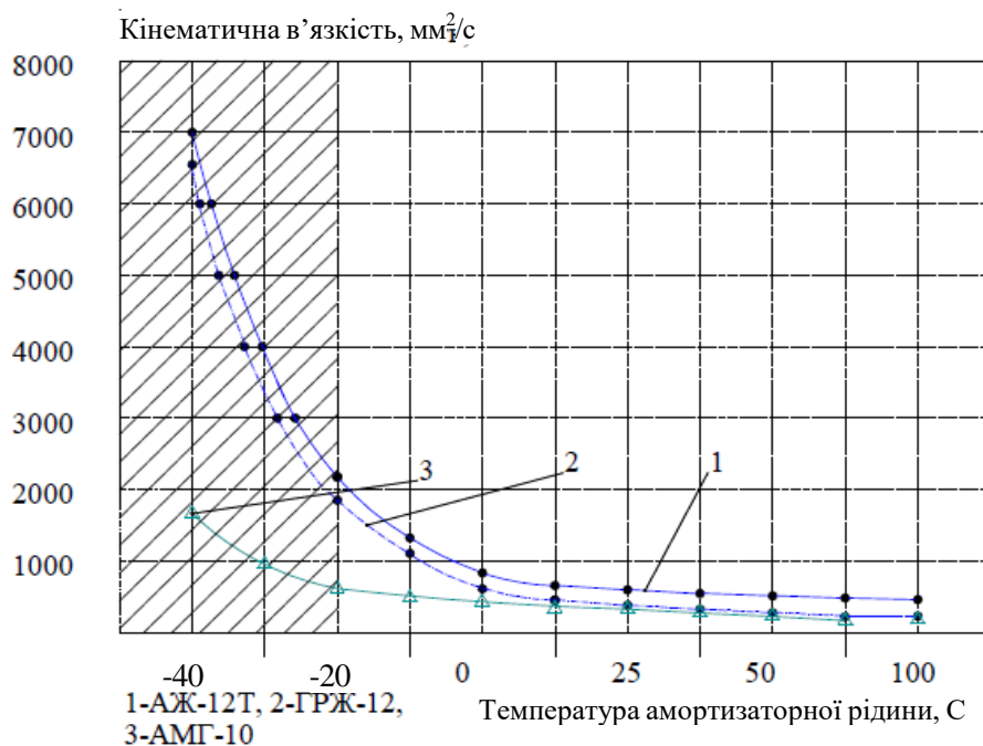
Рисунок 1.7 – Залежність зміни кінематичної в'язкості амортизаторної рідини різних марок від її температури
